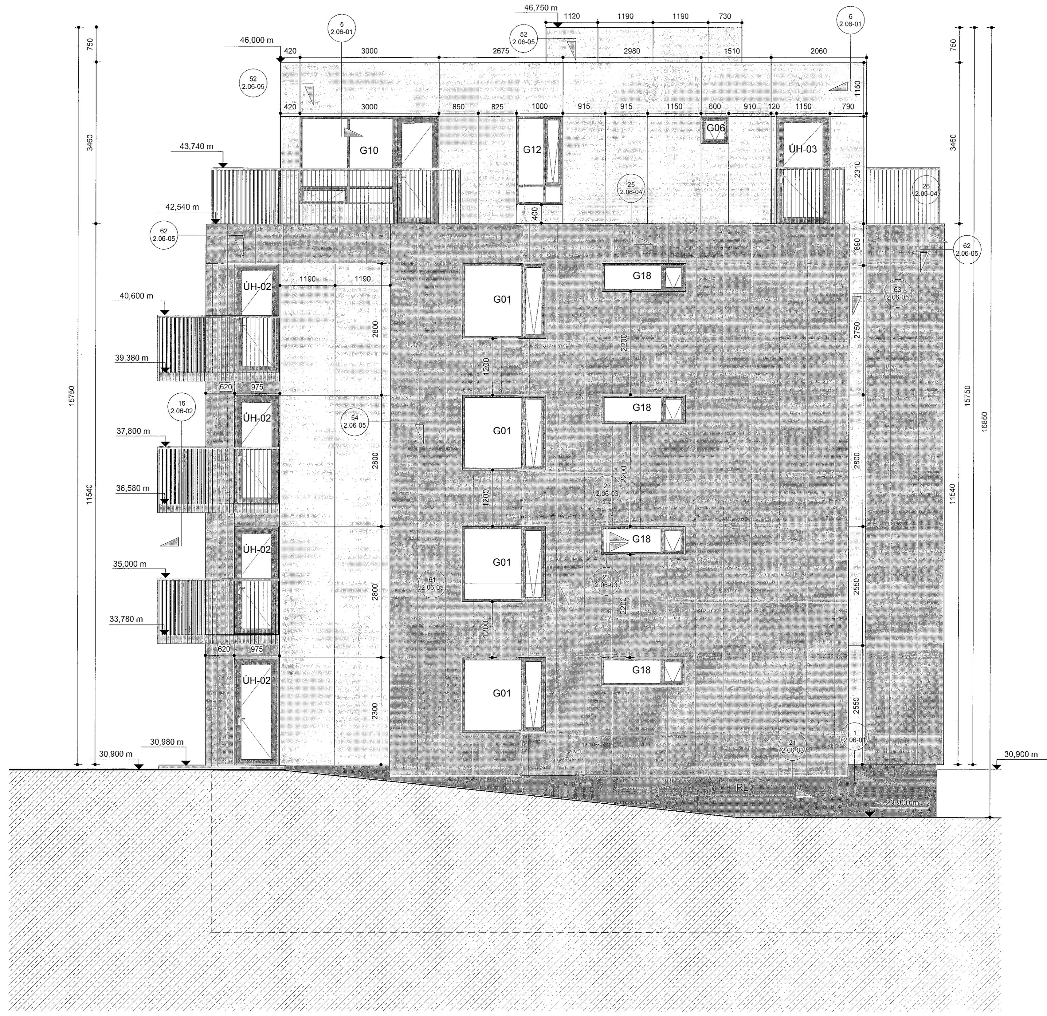
Áshamar 26 ásynd suður verkt. mkv: 1 : 50
