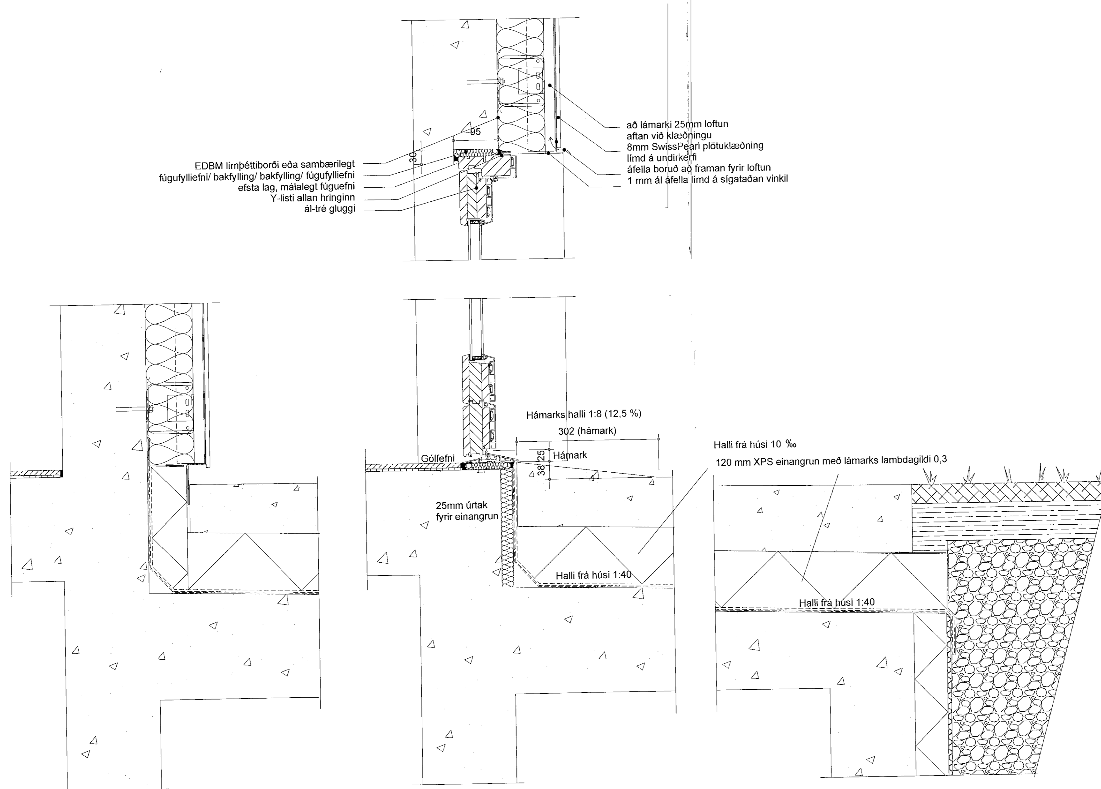
D-71 svalagangsplata að kjallara - mhl.03-04 mkv: 1 : 5
