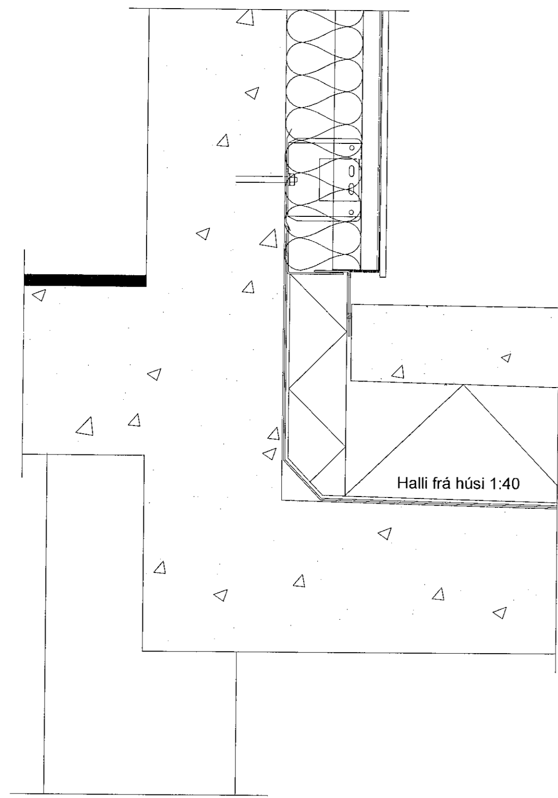
D-73 svalagangsplata ásamt plötum yfir bílakjallara mkv: 1 : 5
