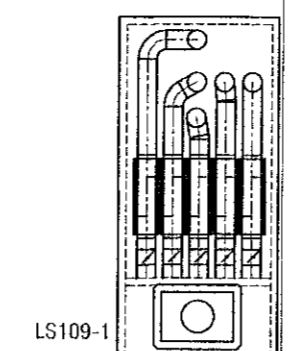
LS109-1 Pakktisari Akst.: 200 l/s við 100 Pa Safkast: 240x100x50 einangurur að innan með 50 mm hjóðþengingardí stöskaplötum. ANUDEC hjóðgildubúskil L=500, á hvest rör.
