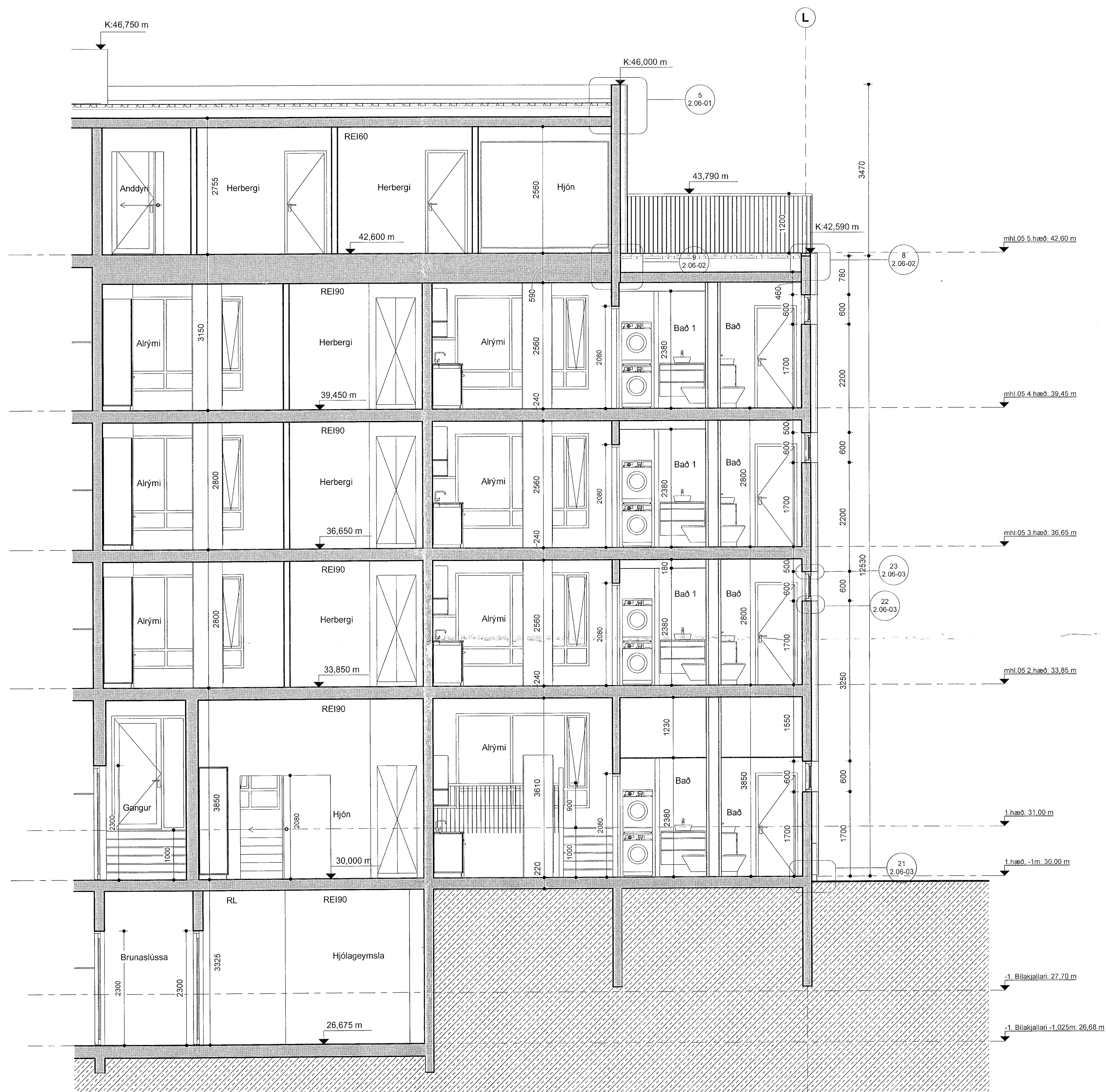
Áshamar 24 mhl.05 - snið g-g - hluti 2 mkv: 1 : 50
