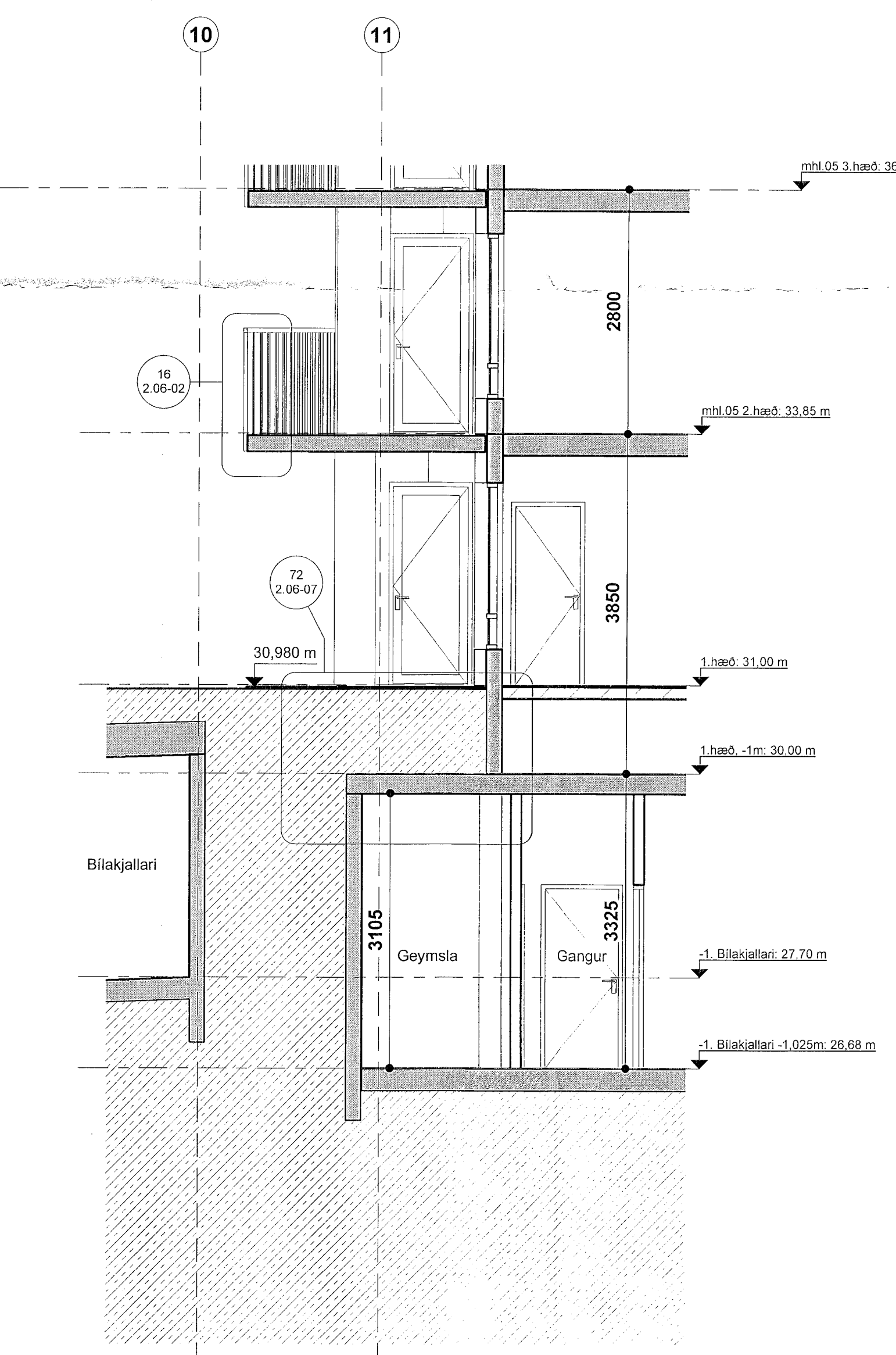
Áshamar 24 mhl.05 - snið - k2-k2 mkv: 1 : 50
