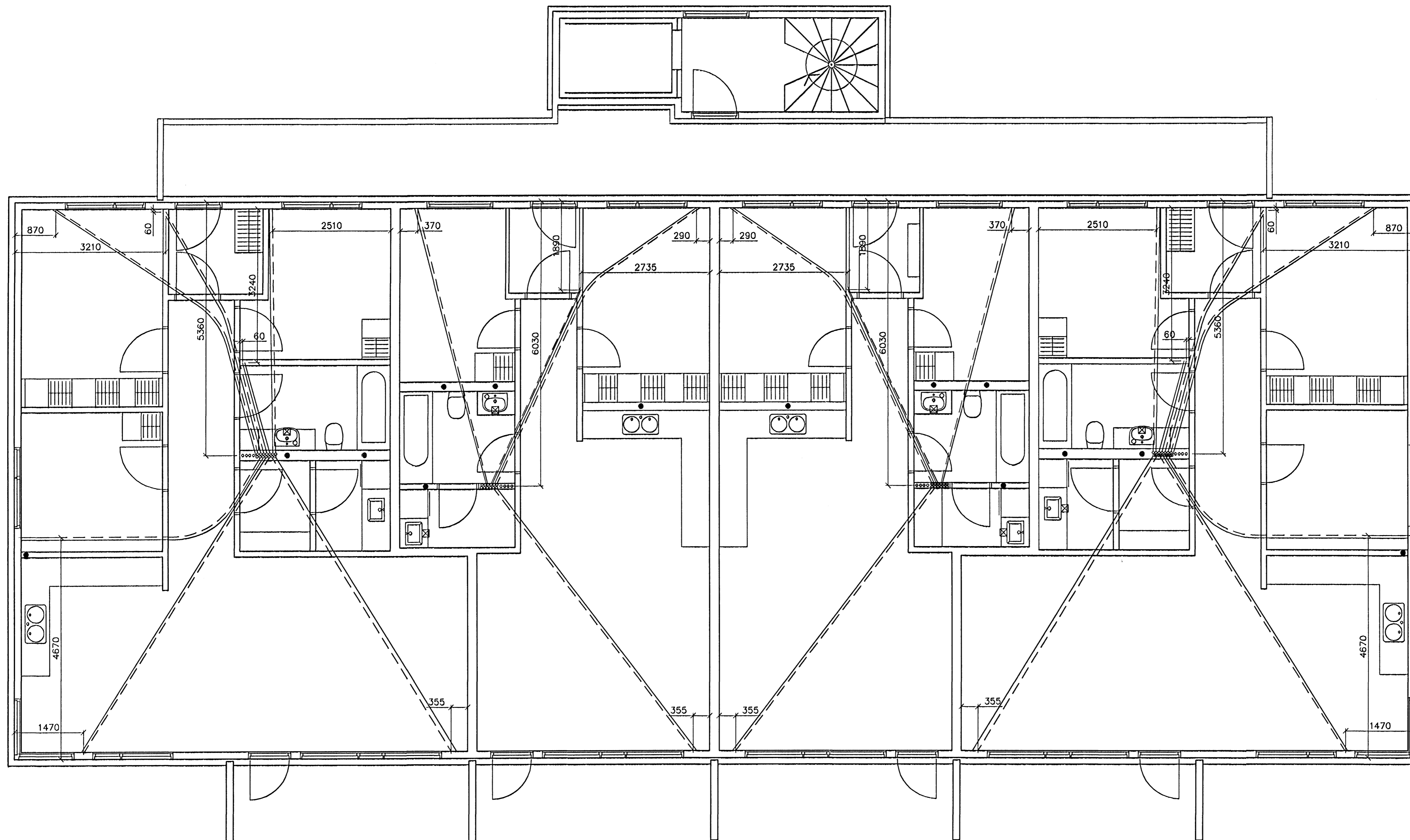
GRUNNMYND 3 HÆÐAR 1:50
