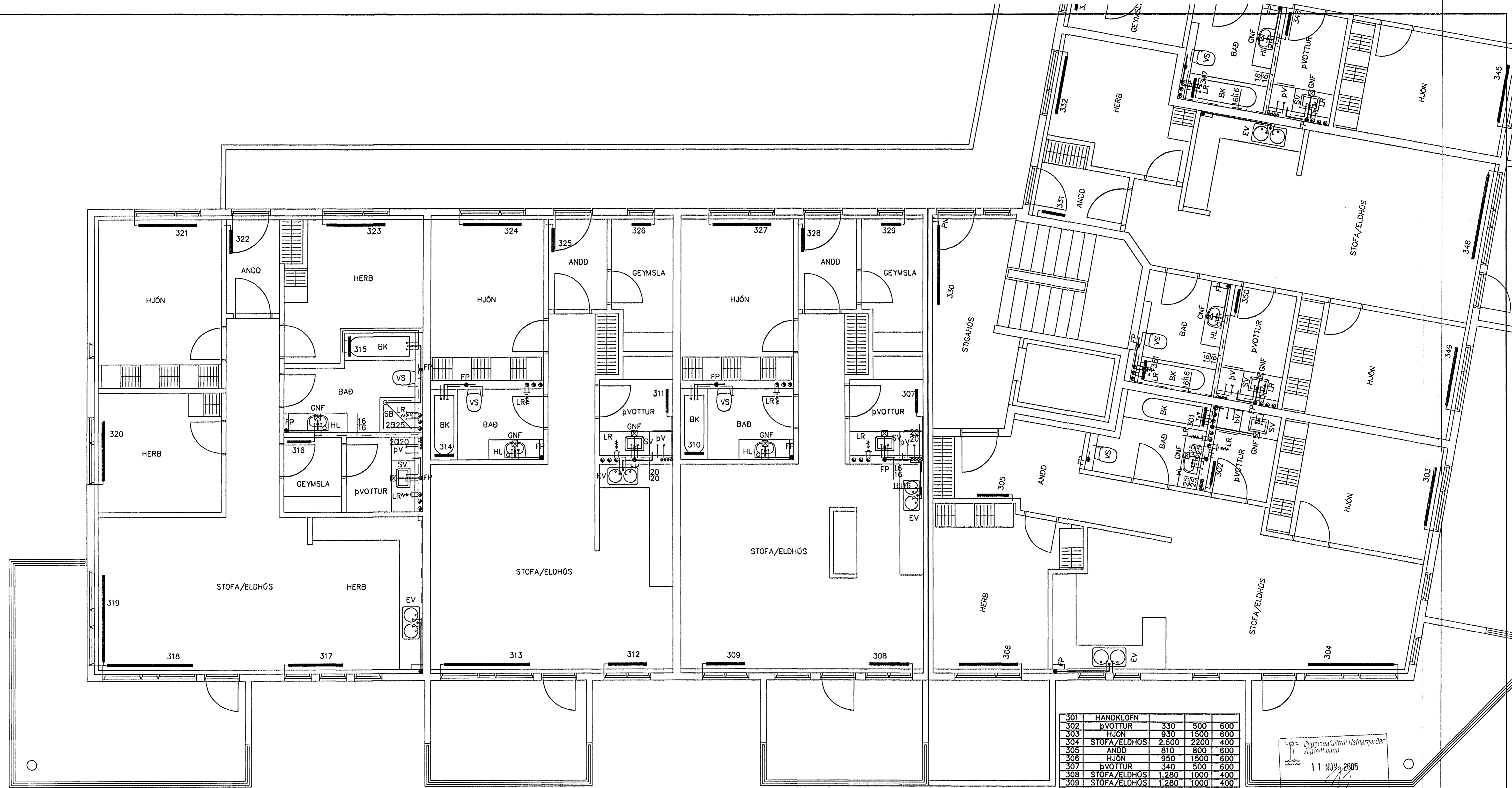
GRUNNMYND 3 HÆÐAR 1:50
