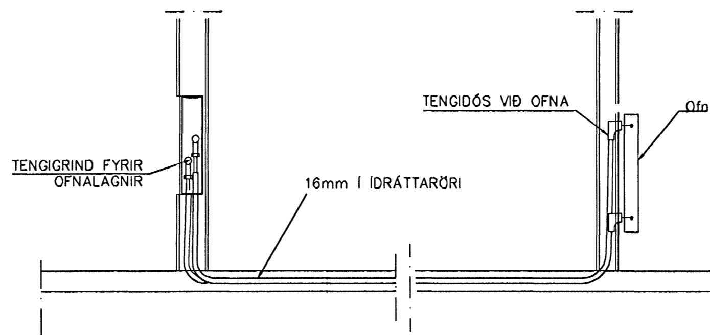
TENGING OFNALAGNALAGNA 1:20
