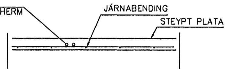
LAGNIR, SNIÐ, 1:20
