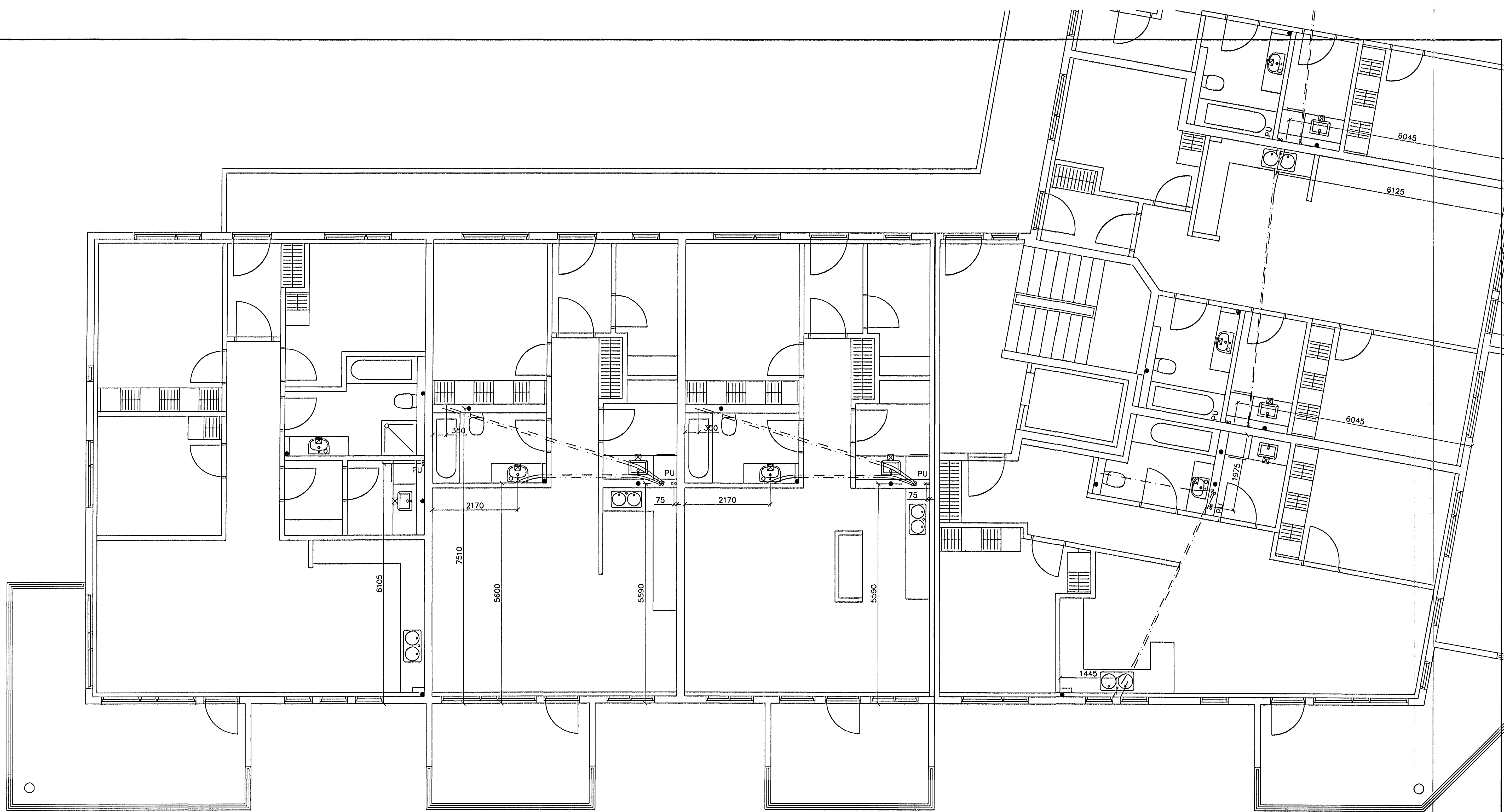
GRUNNMYND 5. HÆÐAR 1:50
