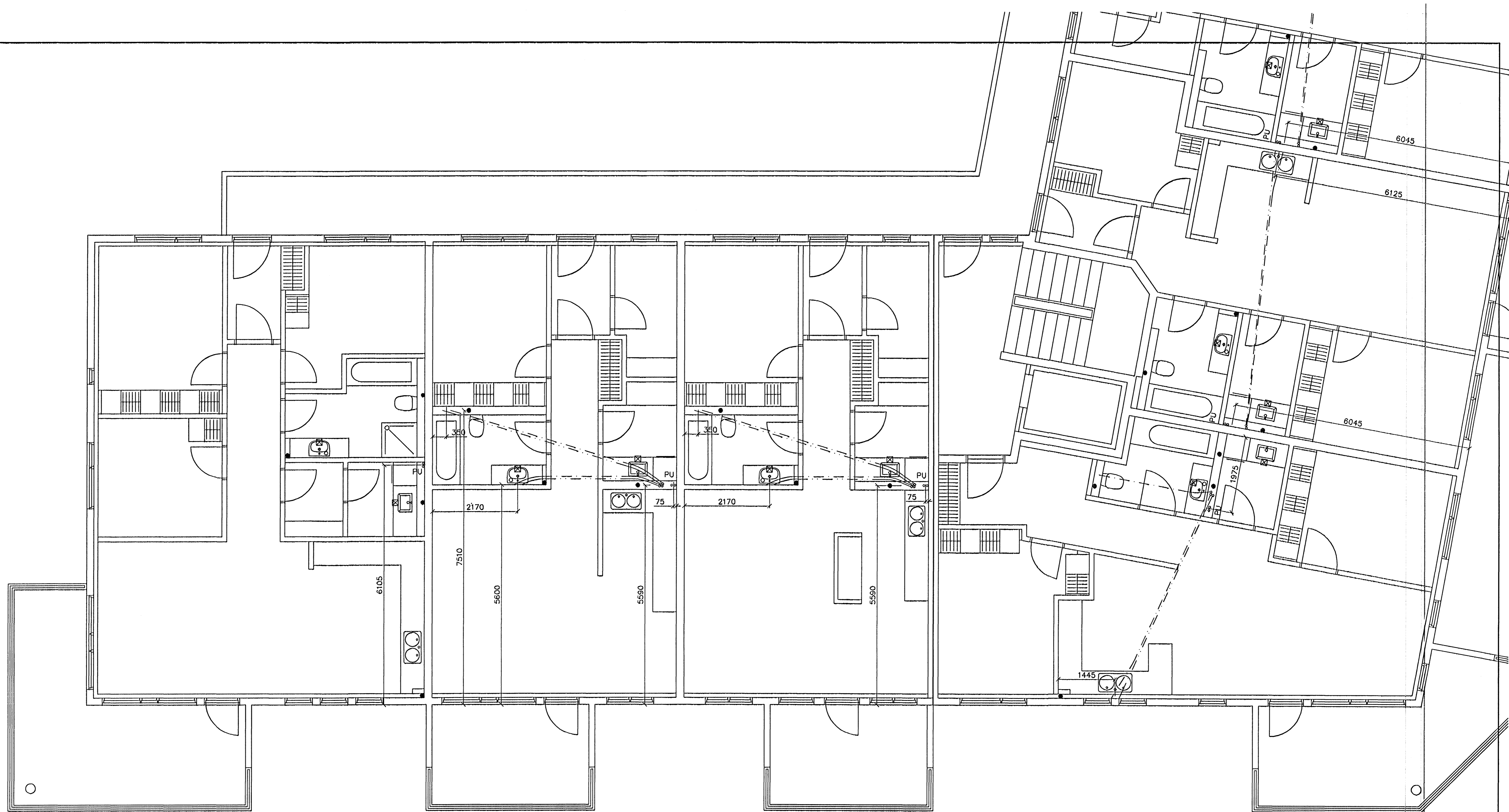
GRUNNMYND 4 HÆÐAR 1:50
