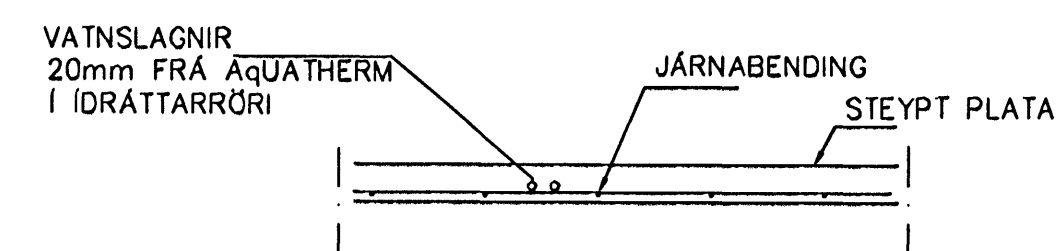
LAGNIR, SNIÐ, 1:20
