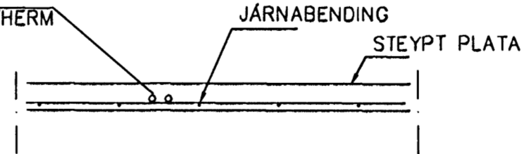
LAGNIR, SNIÐ, 1:20
