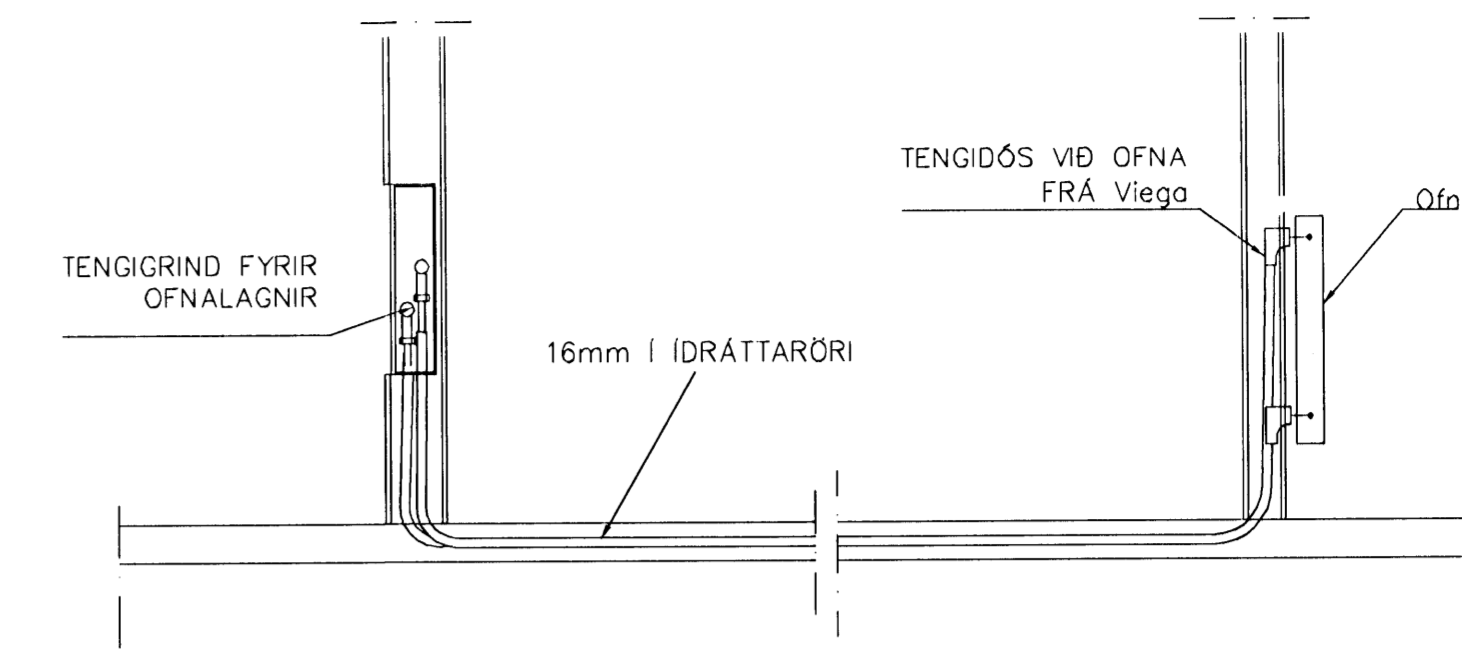
TENGINNIR OFNALAGNALAGNA 1:20
