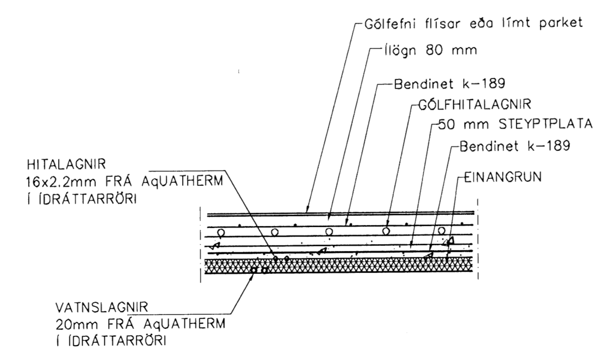
LAGNIR, SNIÐ, 1:20
