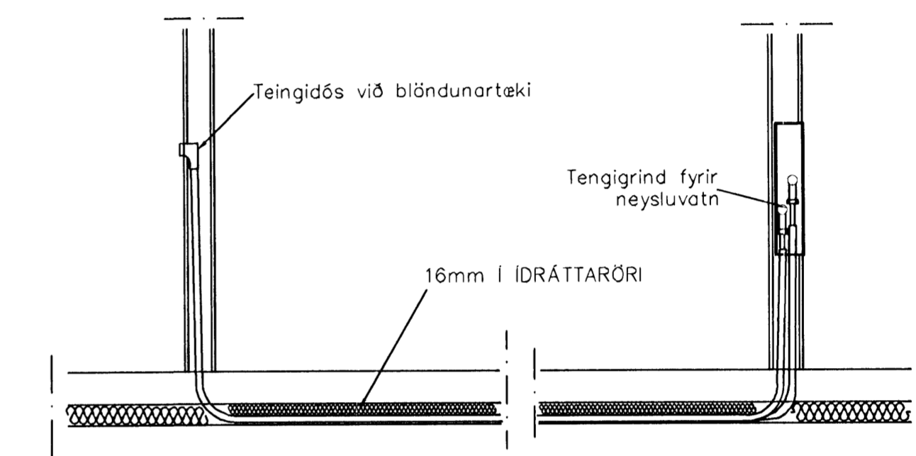
TENGINNIR NEYSLUVATNSLAGNA 1:20
