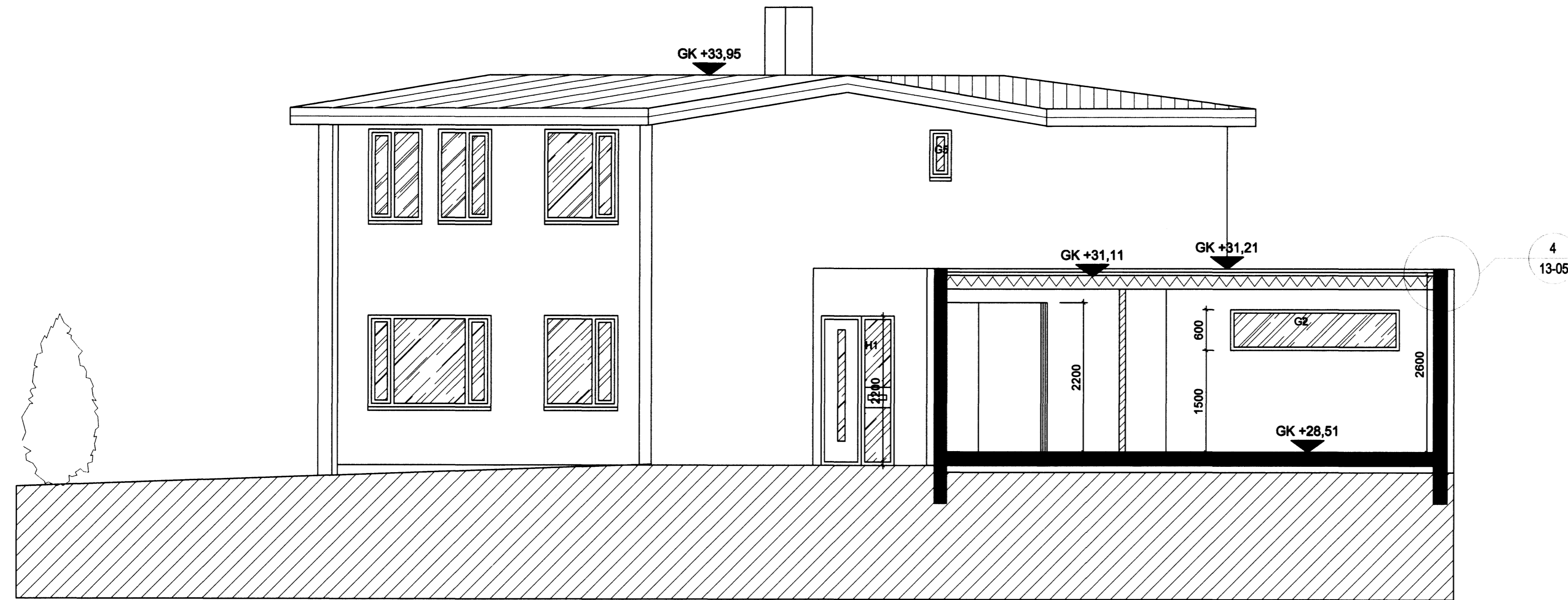
SNEIDING X-X 1:50
