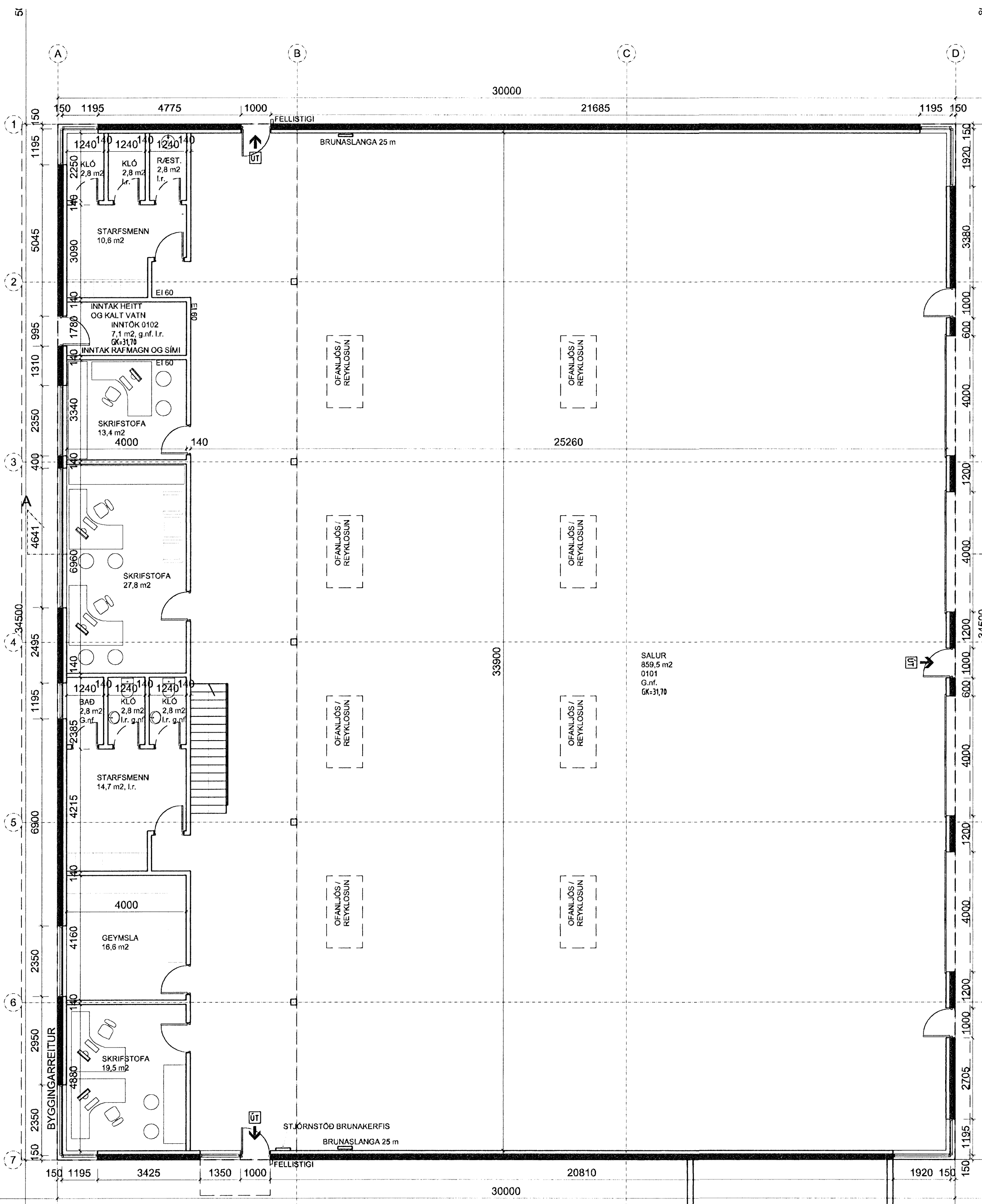
GRUNNMYND 1. HÆÐ 1/100
