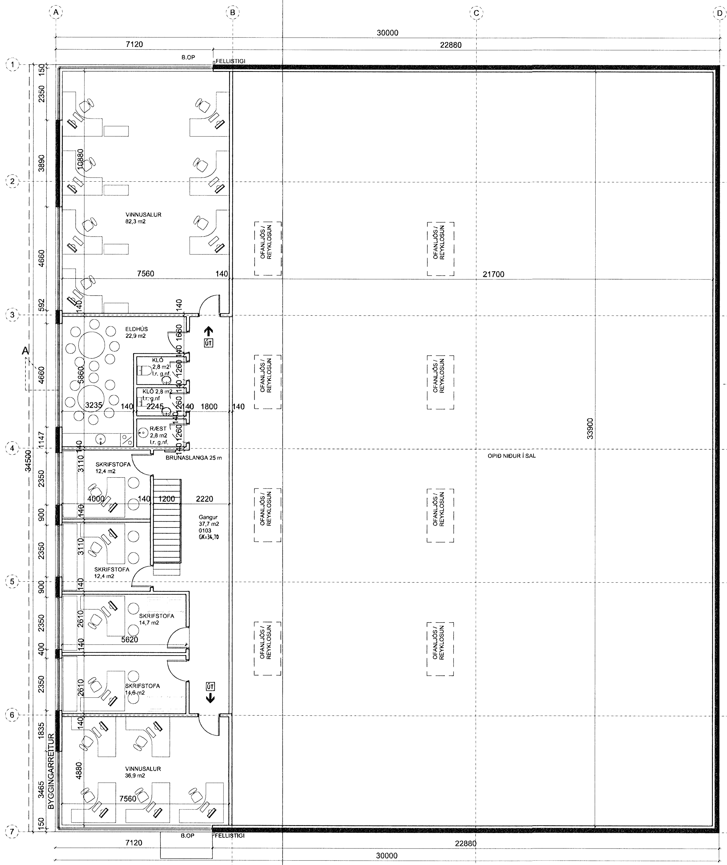
GRUNNMYND MILLIPALLUR 1/100
