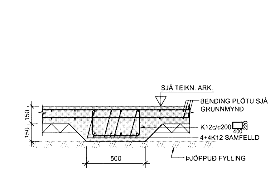
4 SNID 1:20
