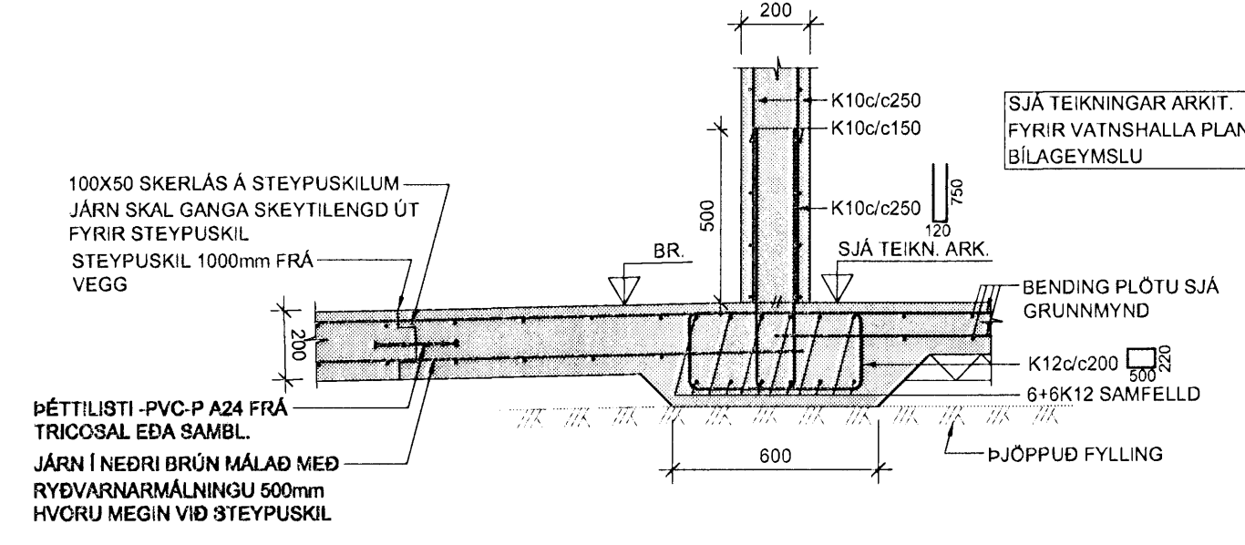
6 SNID 1:20
