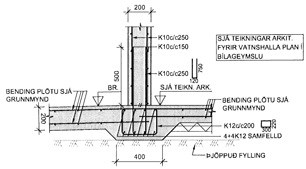
2 SNID 1:20
