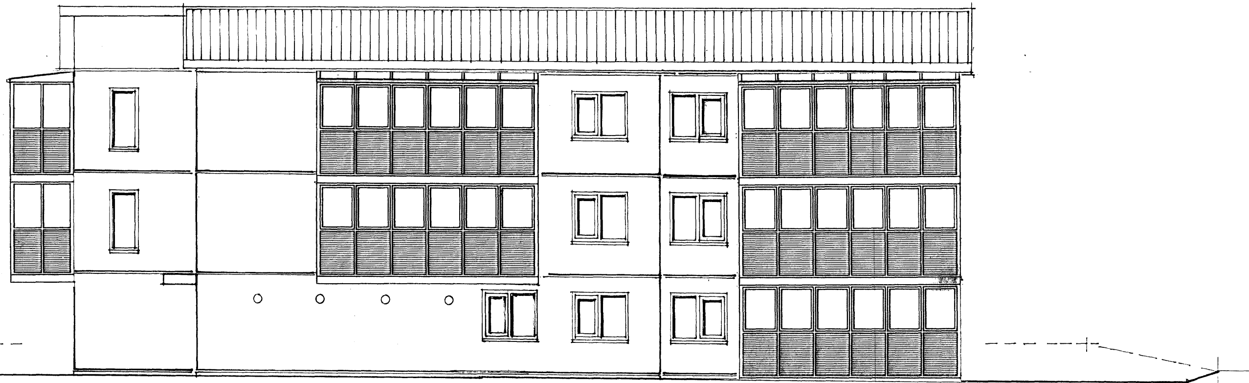
ÚTLIT SUÐVESTUR MKV. 1:100
