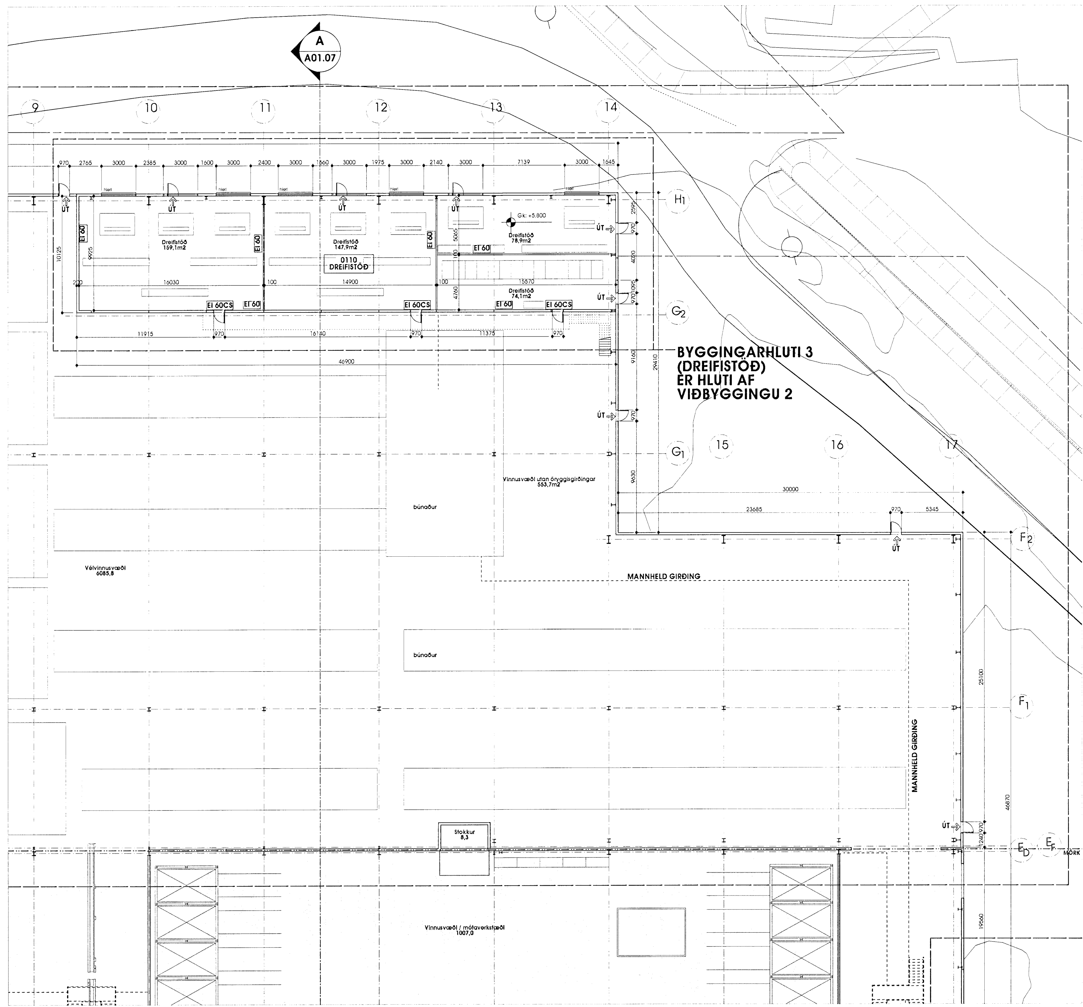
1 GRUNNMYND 1.HÆÐ - VIÐBYGGING 2 - HLUTI 2 / BYGGINGARHLUTI 3 - DREIFISTÖÐ mkv. 1:200
