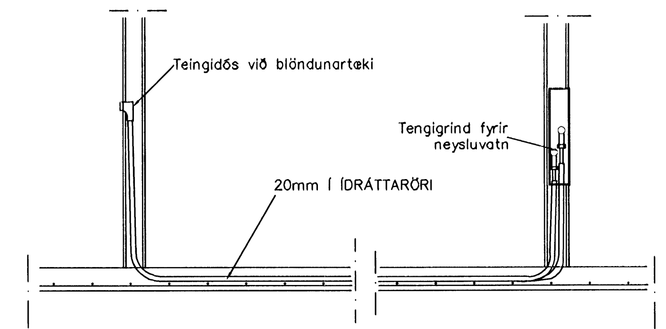
TENING NEYSLUVATNSLAGNA 1:20
