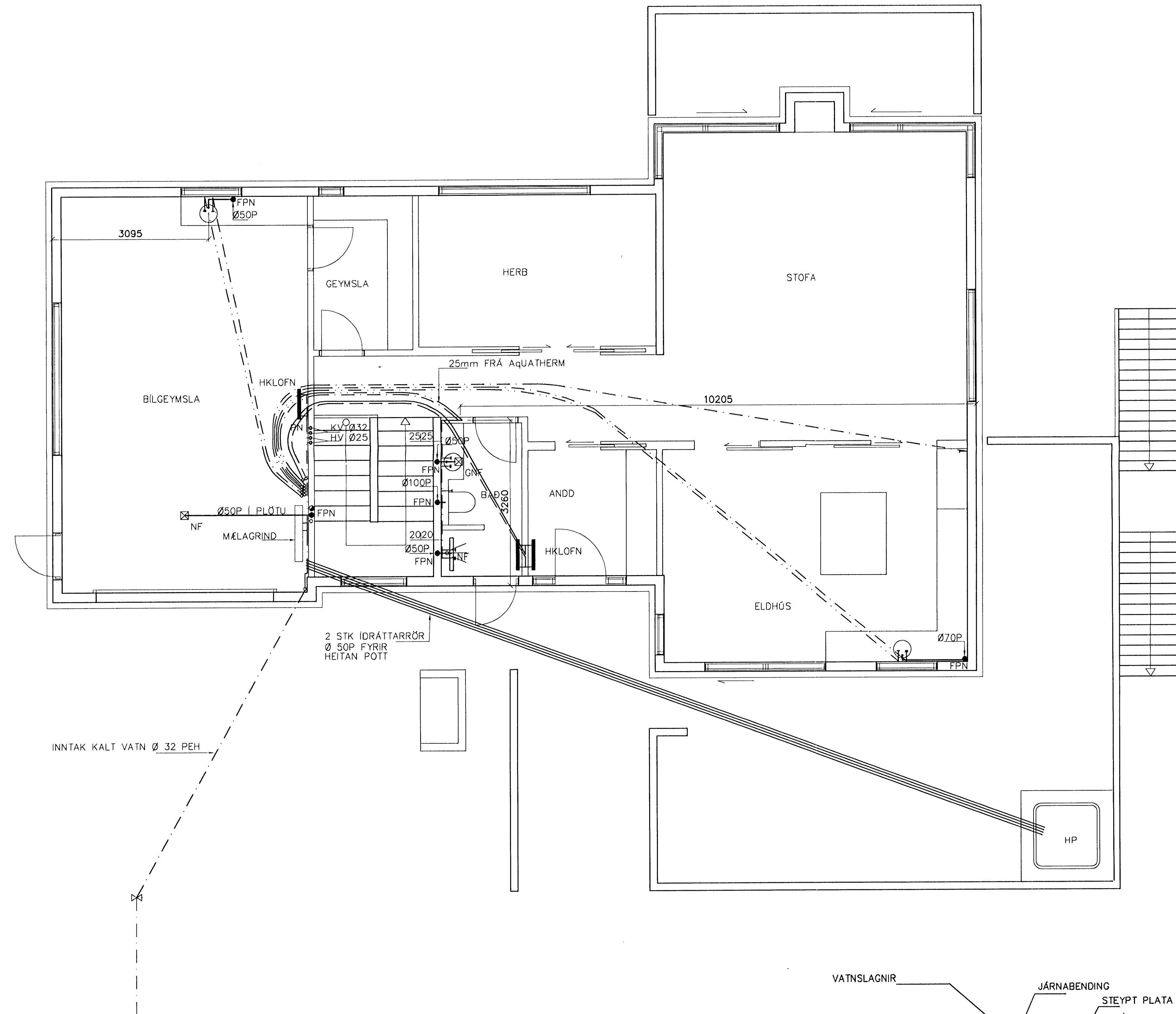
GRUNNMYND 2 HÆÐAR 1:50
