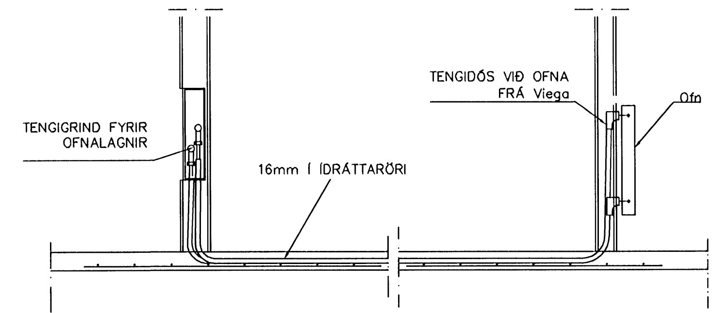
TENING OFNALAGNALAGNA 1:20
