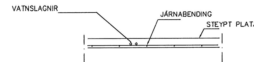
LAGNIR, SNÍÐ, 1:20
