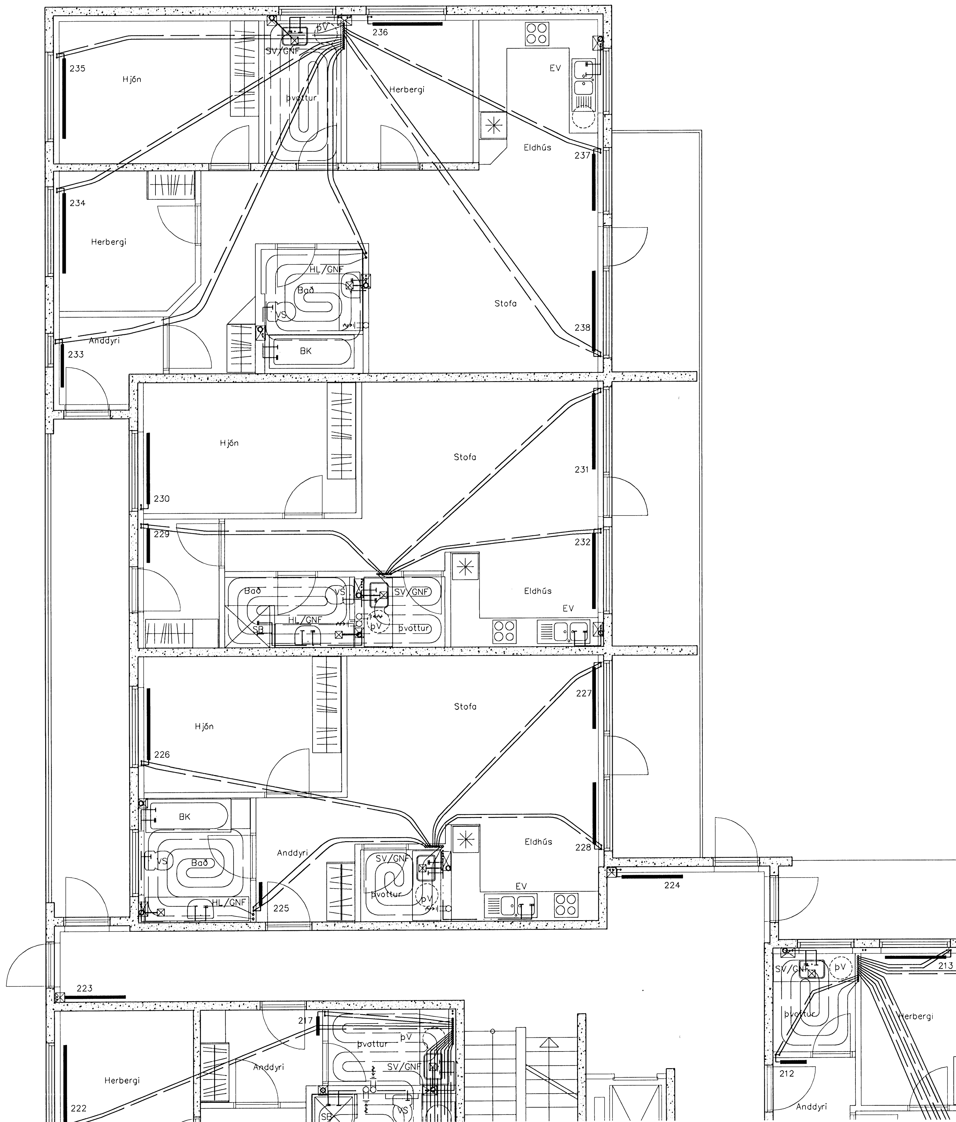
Lagnir 2. hæð, 1:50
