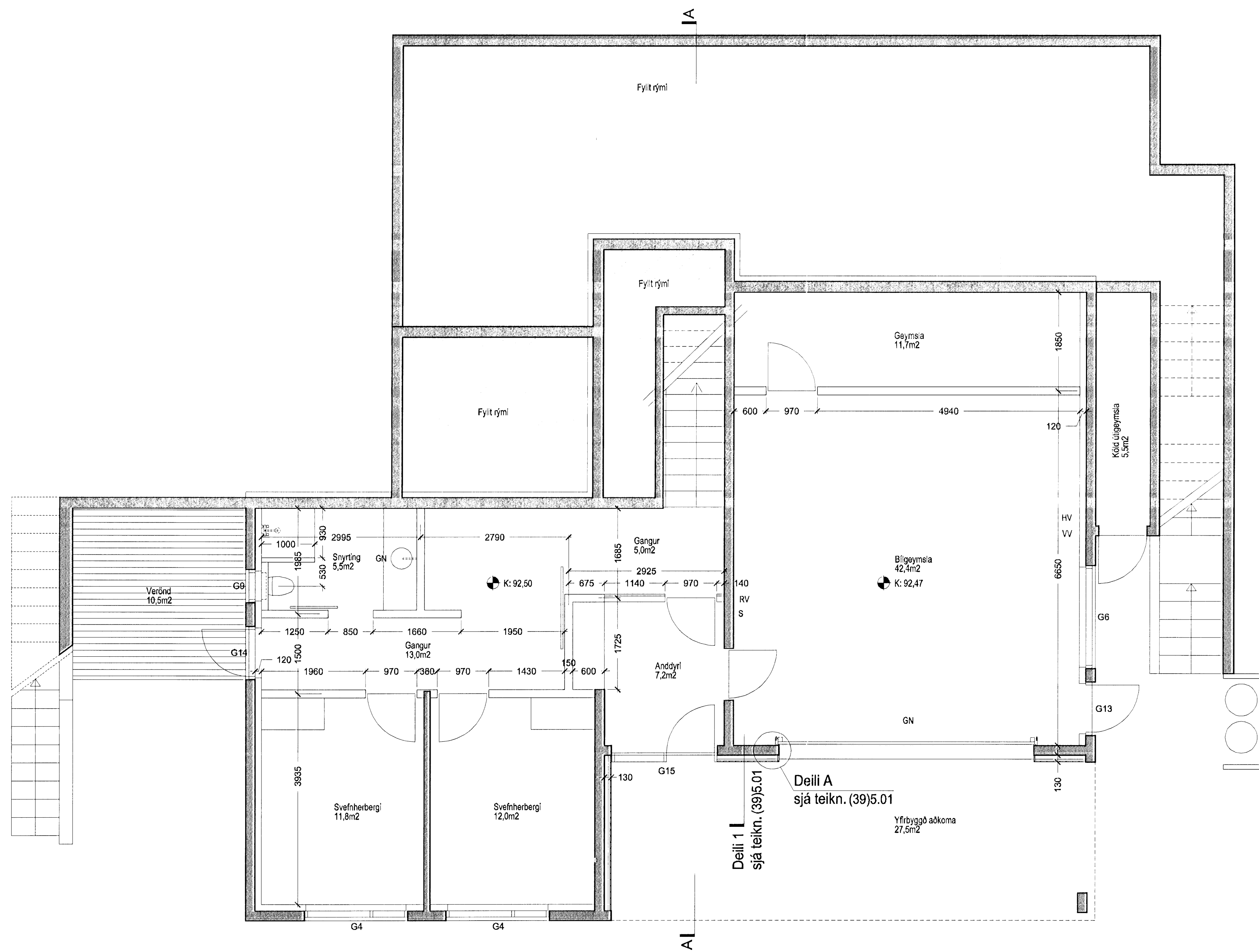
GRUNNMYND 1. HÆÐAR í mkv. 1:50
