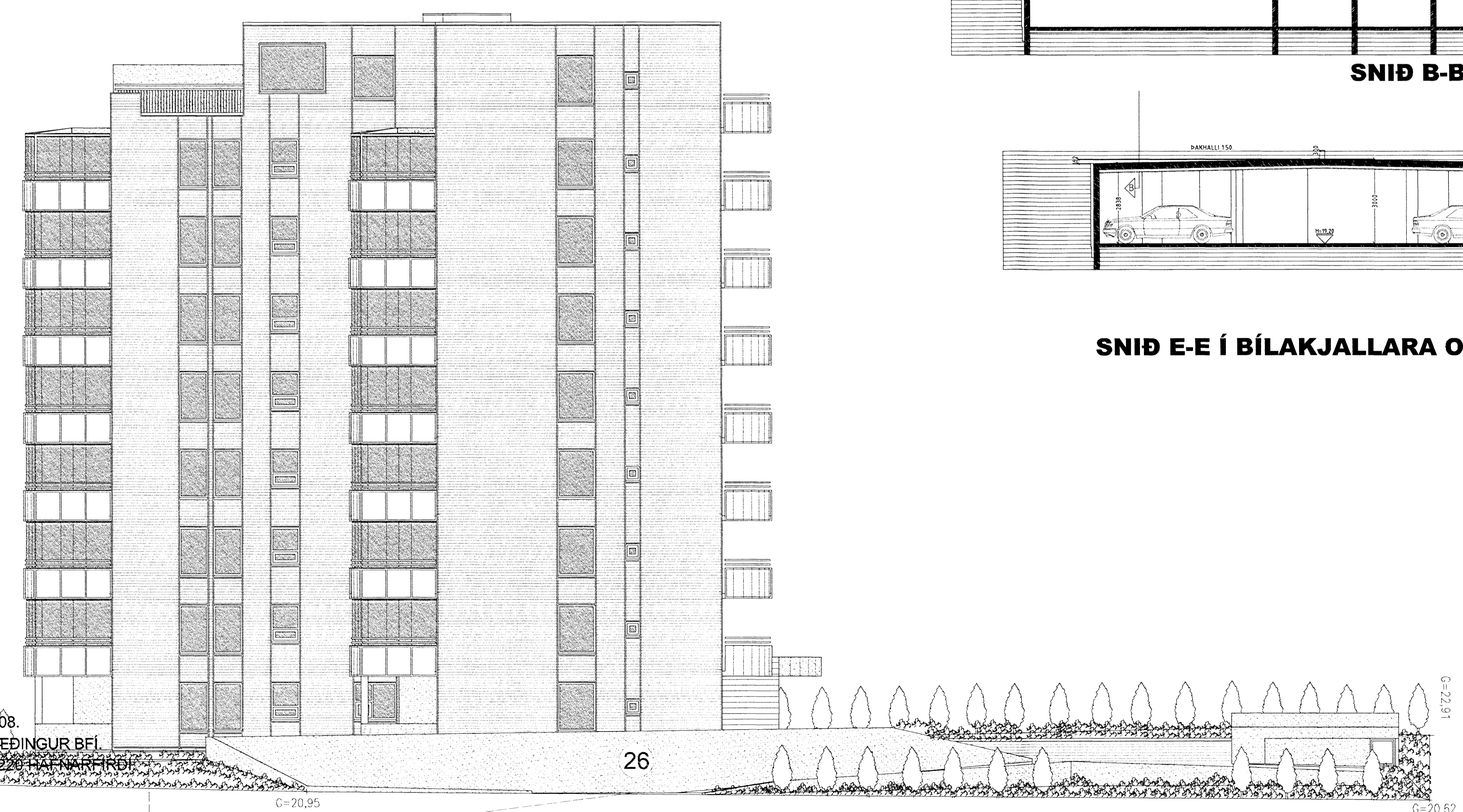
ÚTLIT AUSTUR MKV. 1:100.
