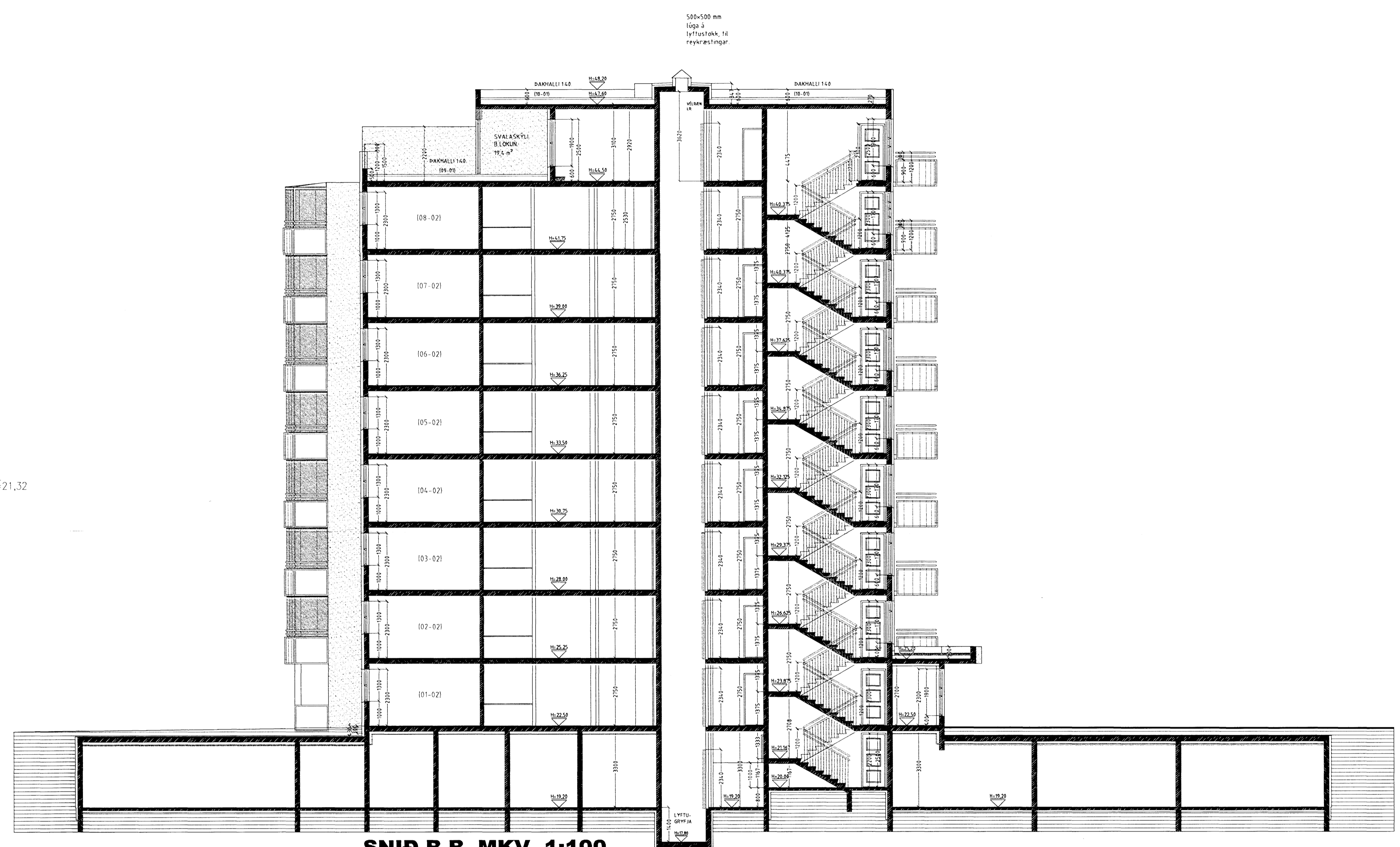
SNID B-B MKV. 1:100.
