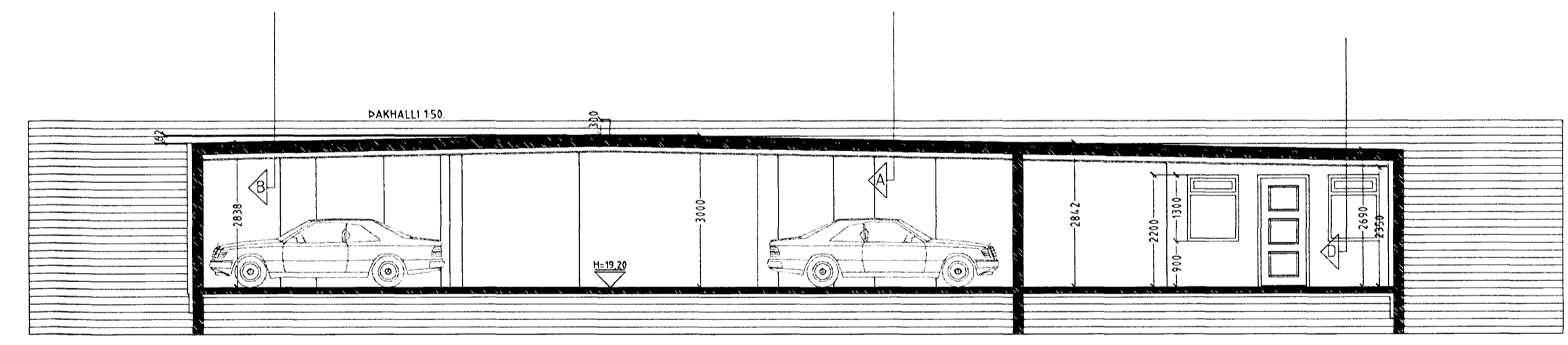
SNID B-B MKV. 1:100.
