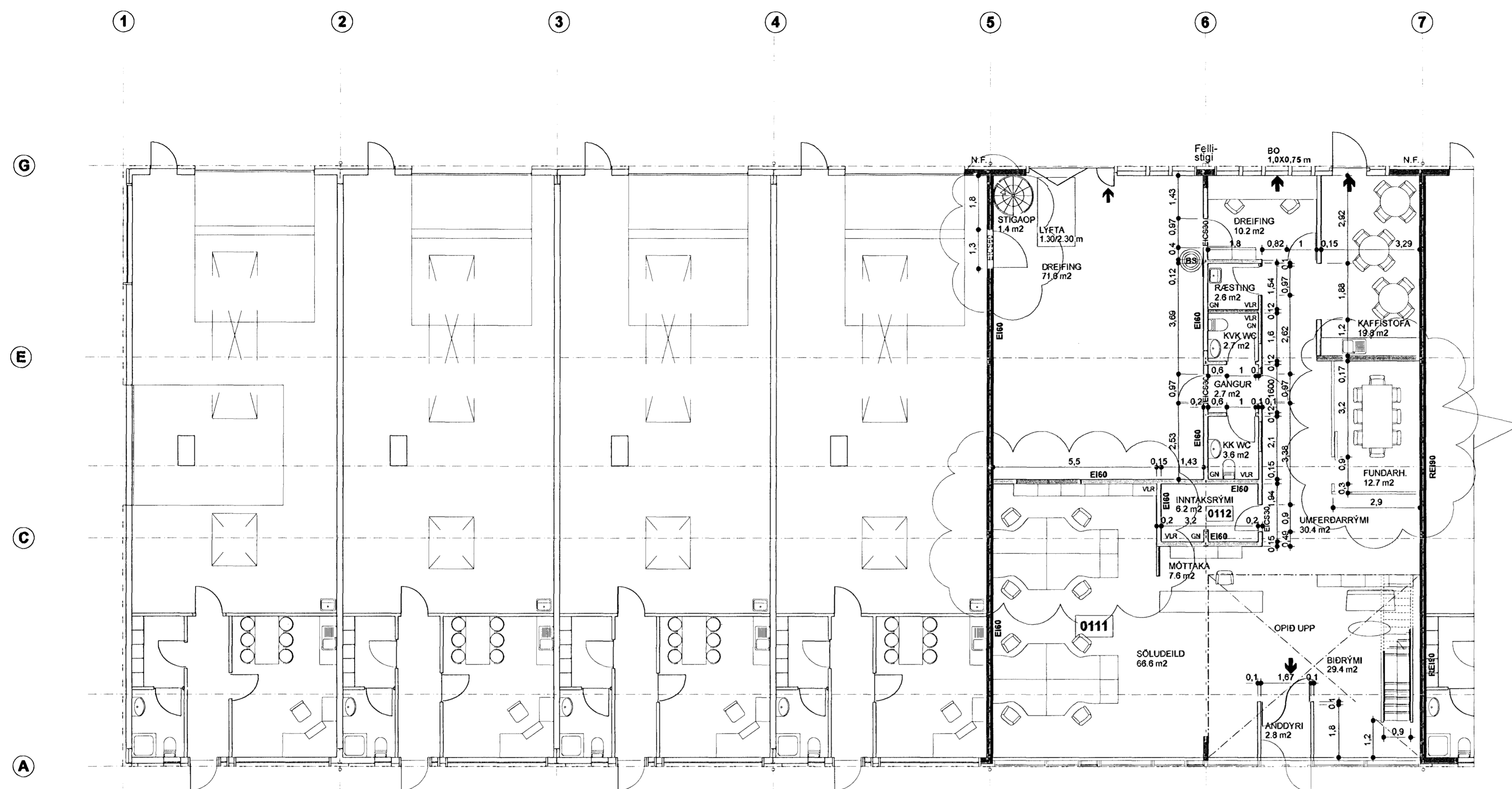
1. HÆÐ (1)
