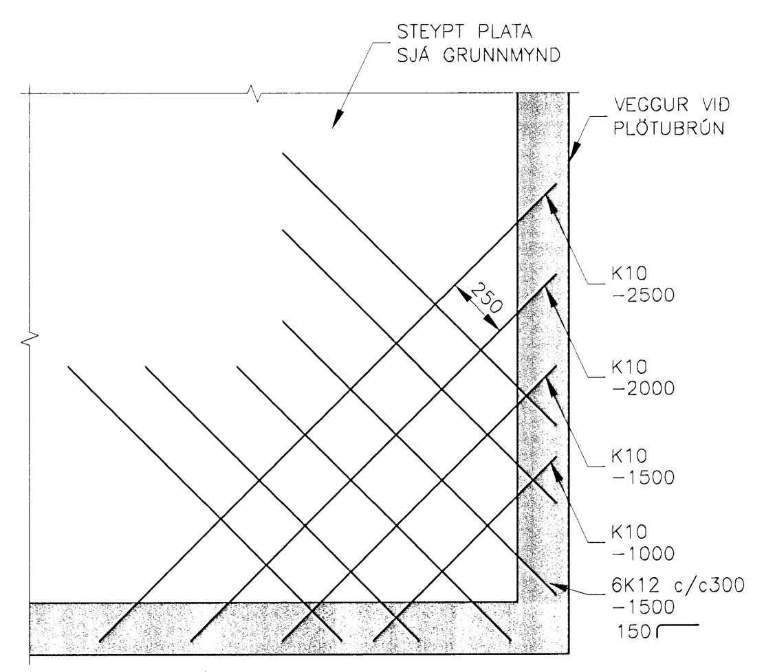
D52 JÁRNBENDING Í PLÖTUHORN MKV. 1
