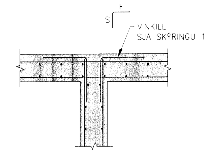
D02 DÆMIGERÐ JÁRNBENDING Í SAMSEYPTUM VEGGJA OG PLATNA – LÖÐRÉTT SNID MKV. 1
