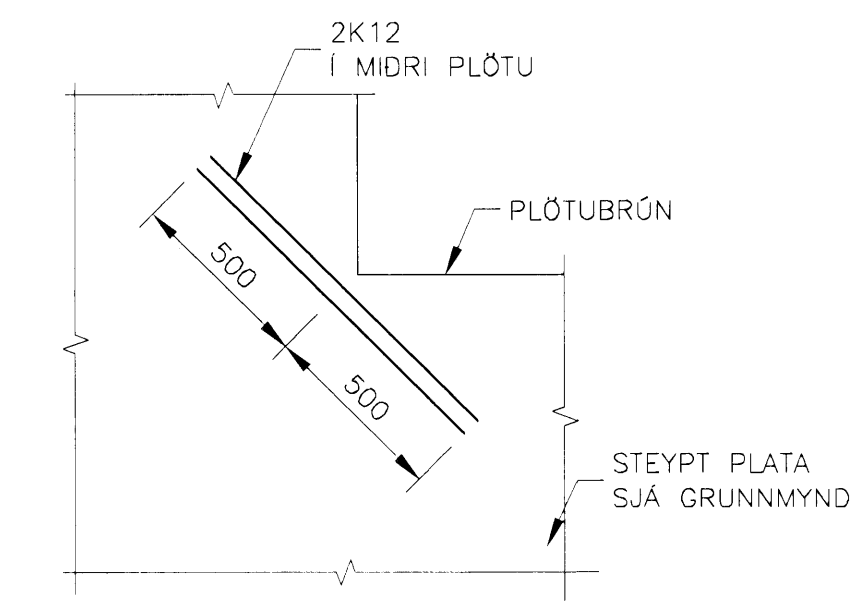
D51 JÁRNBENDING Í PLÖTUHORN MKV. 1
