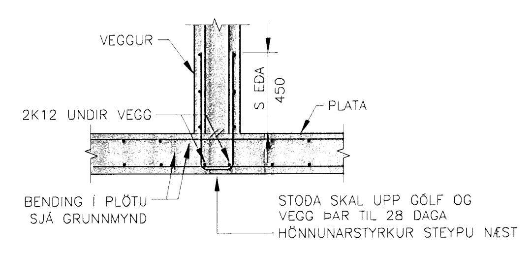
D02 DÆMIGERÐ JÁRNBENDING Í SAMSEYPTUM VEGGJA OG PLATNA – LÖÐRÉTT SNID MKV. 1
