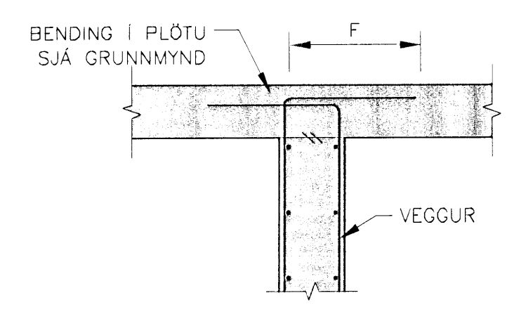
D02 DÆMIGERÐ JÁRNBENDING Í SAMSEYPTUM VEGGJA OG PLATNA – LÖÐRÉTT SNID MKV. 1
