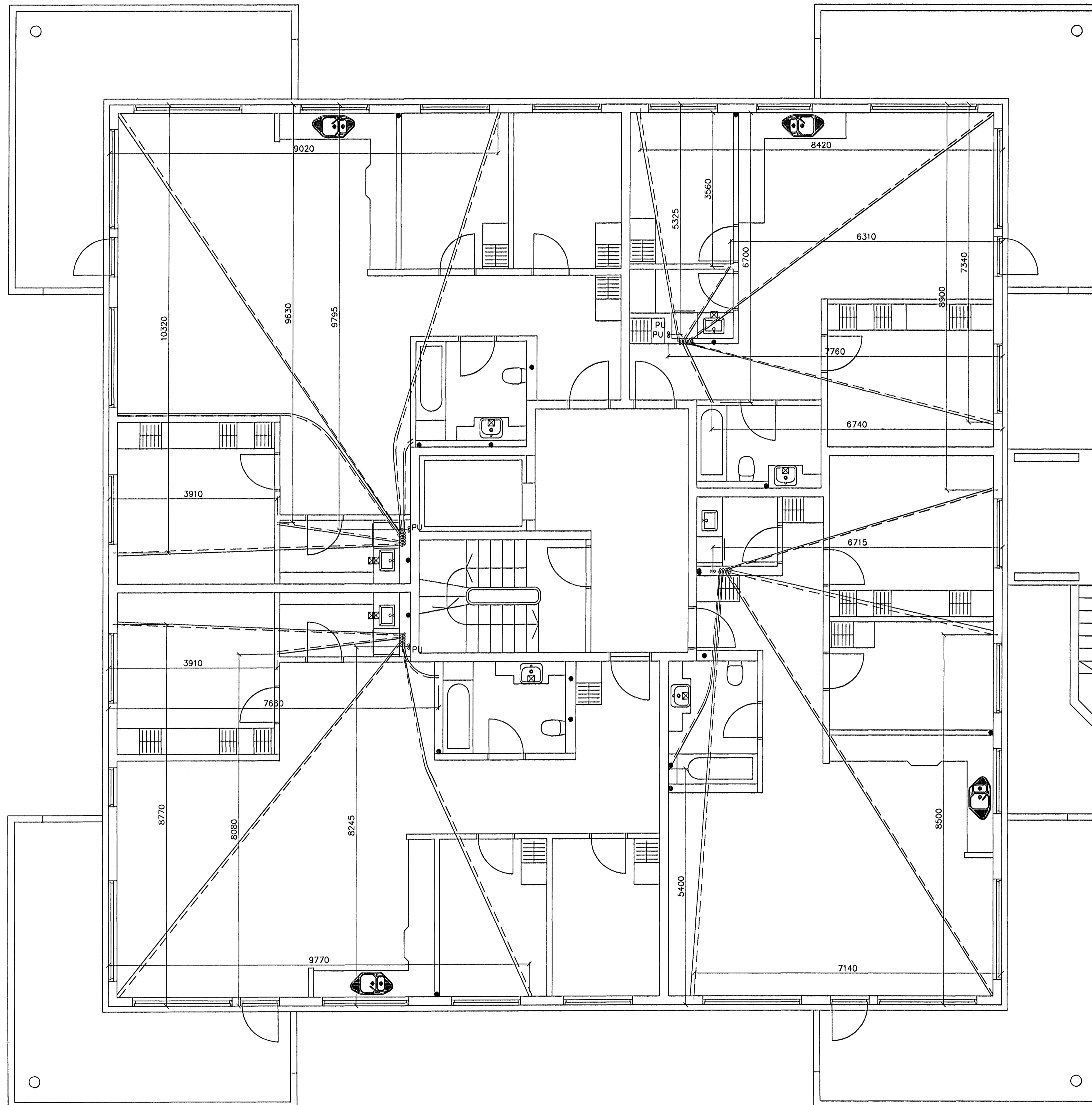
GRUNNMYND 3 HÆÐAR 1:50
