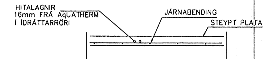
LAGNIR, SNIÐ, 1:20
