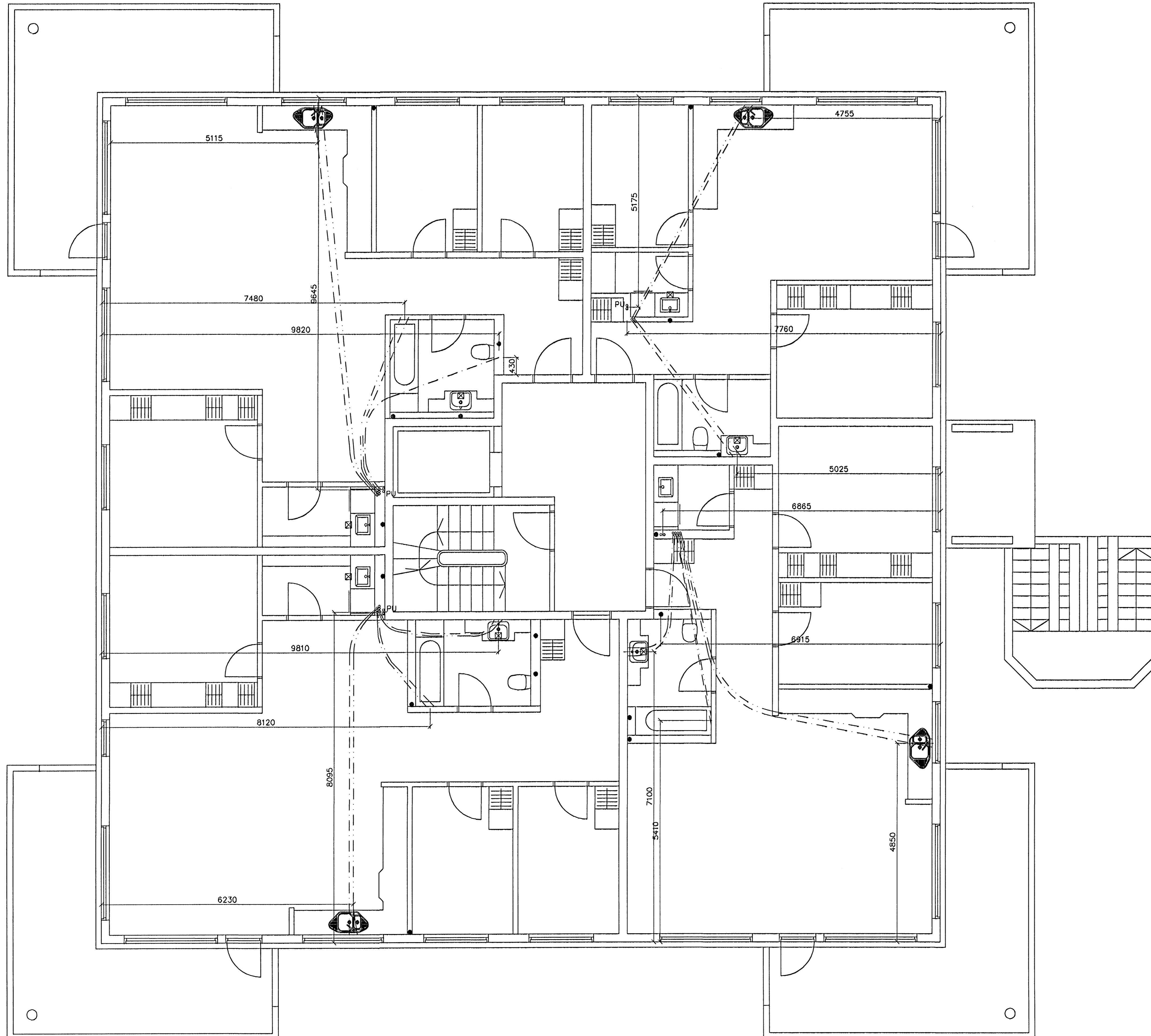
GRUNNMYND 3 HÆÐAR 1:50
