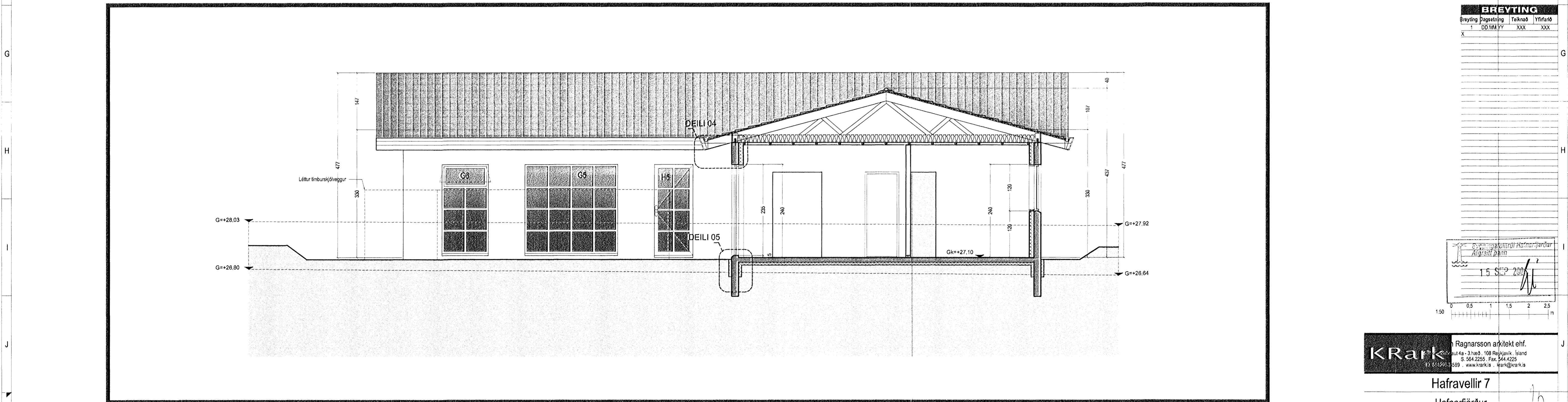
Snið 2 1:50
