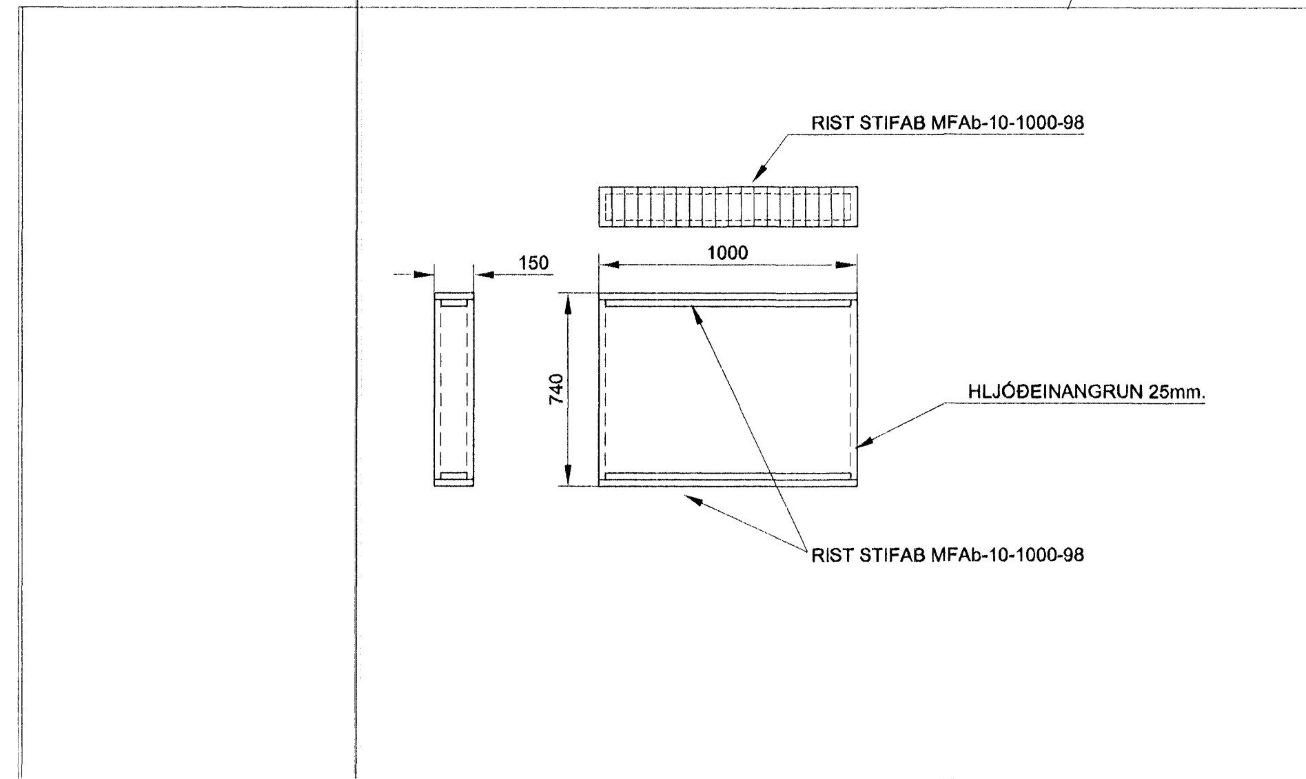
DÆMIGERT HLJÓÐEYFIBOX MILLI HÆÐA 1:20
