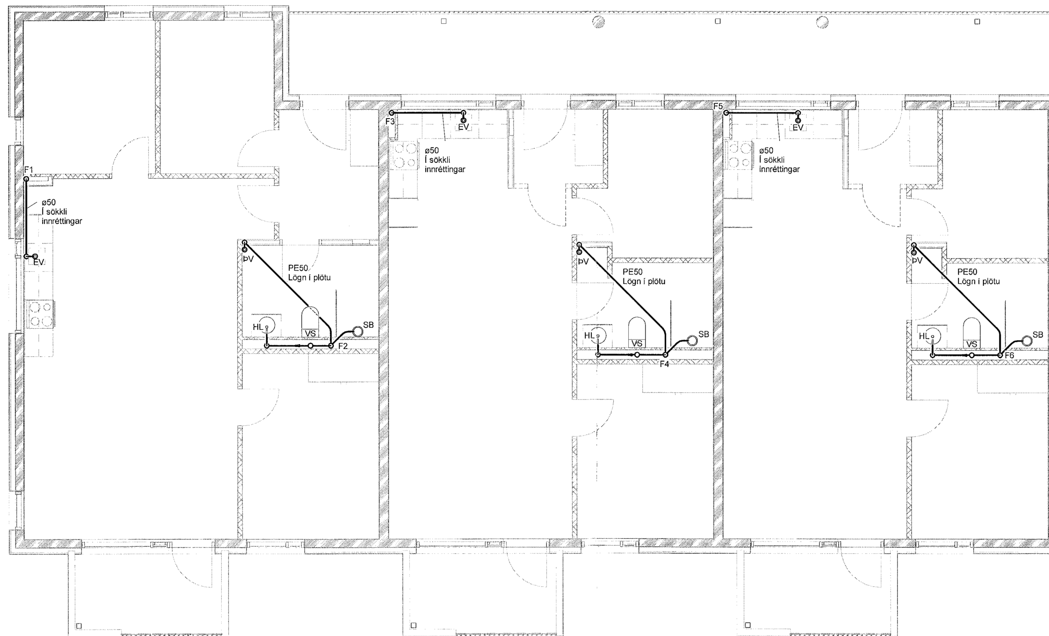
1 4. hæð - 1 1 : 50
