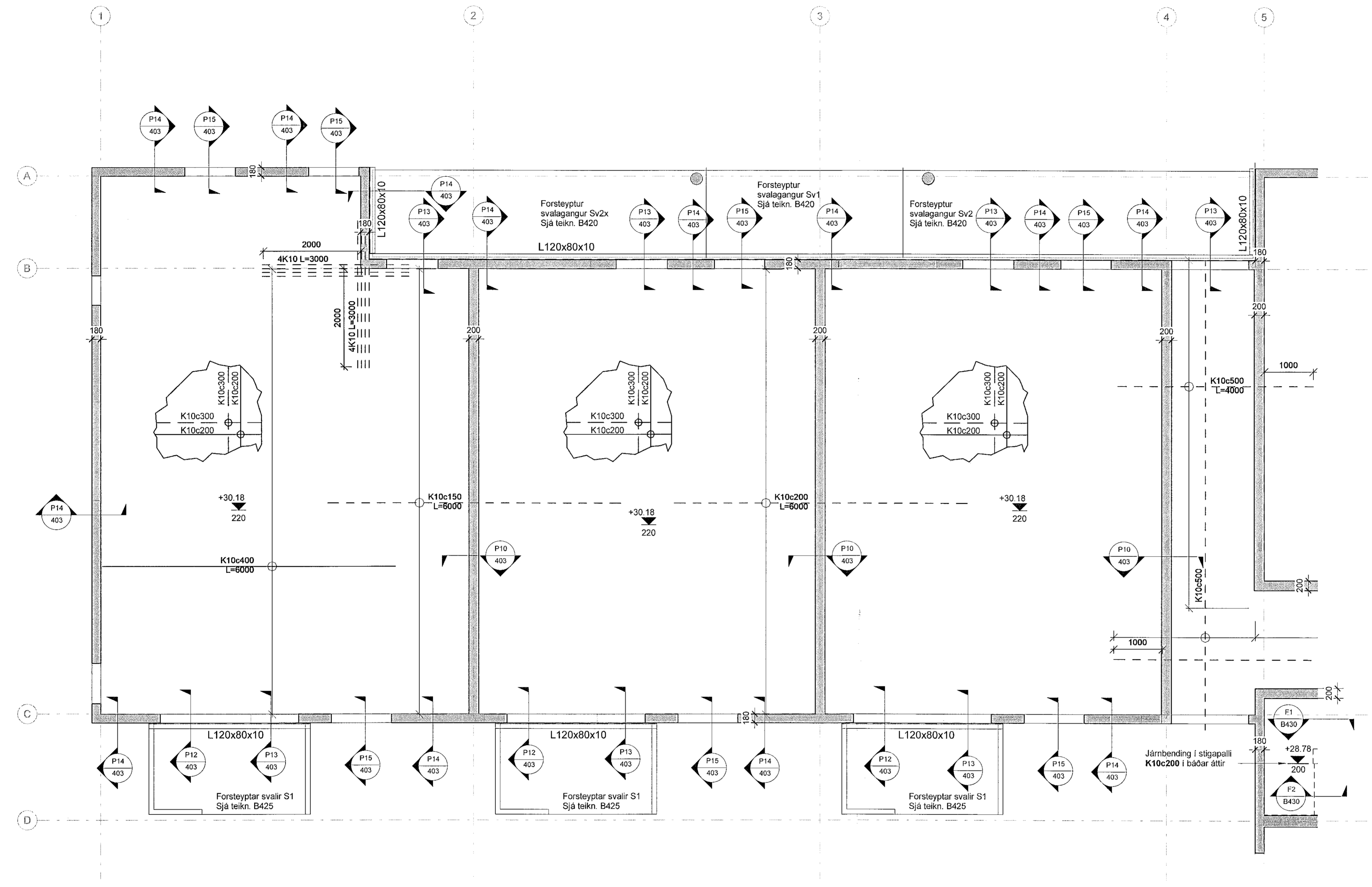
1 1. hæð - Loftaplata og veggir - 1/3 1 : 50
