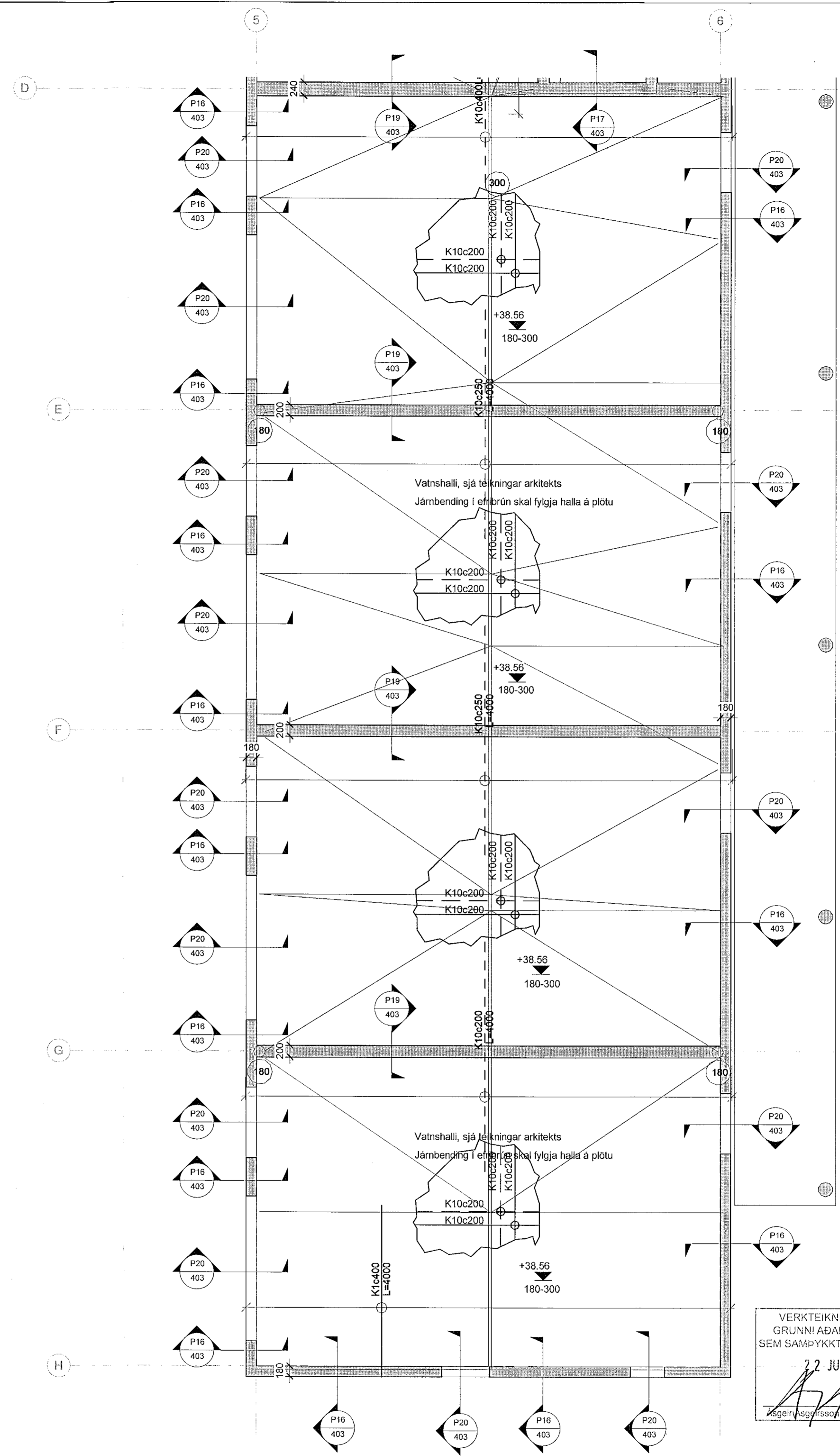
2 4. hæð - Þakplata og veggir - 3/3 1 : 50
