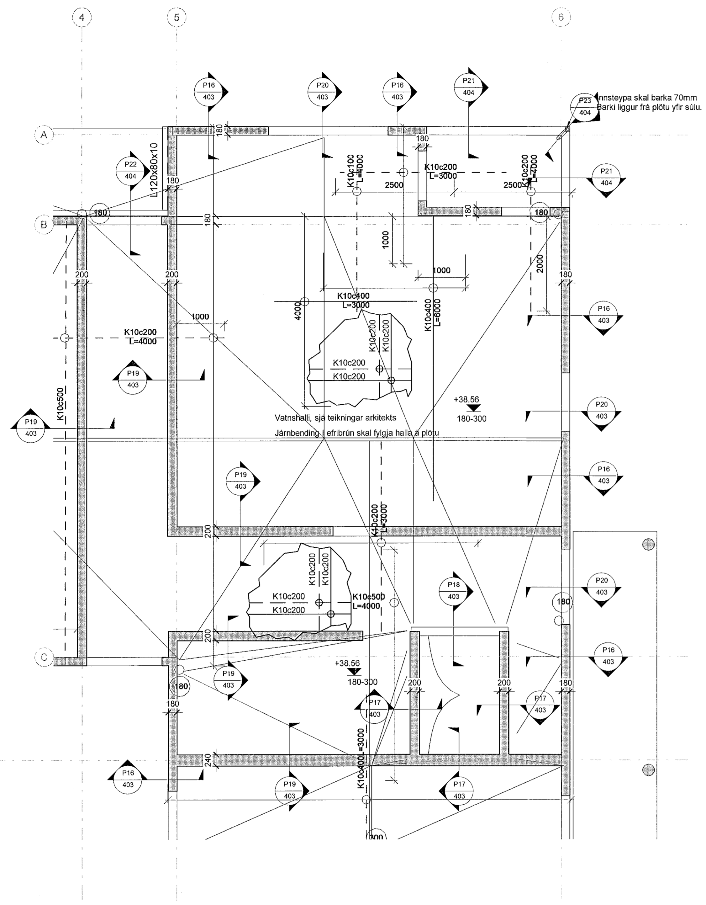
1 4. hæð - Þakplata og veggir - 2/3 1 : 50
