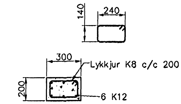
Súla S.1 1:20 1-05
