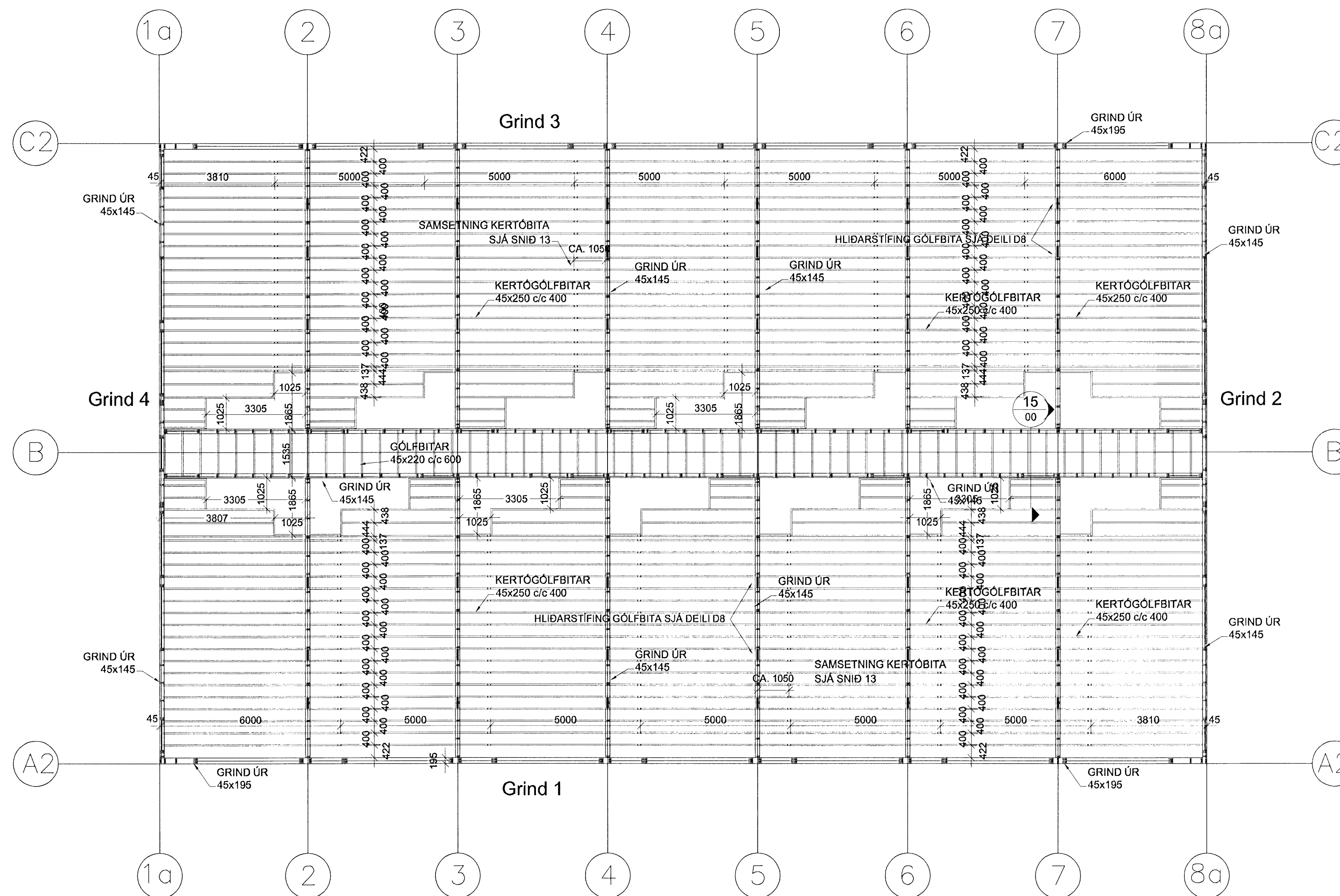
MILLIGÓLF-GÓLFBITAR GRUNNMYND 1:100
