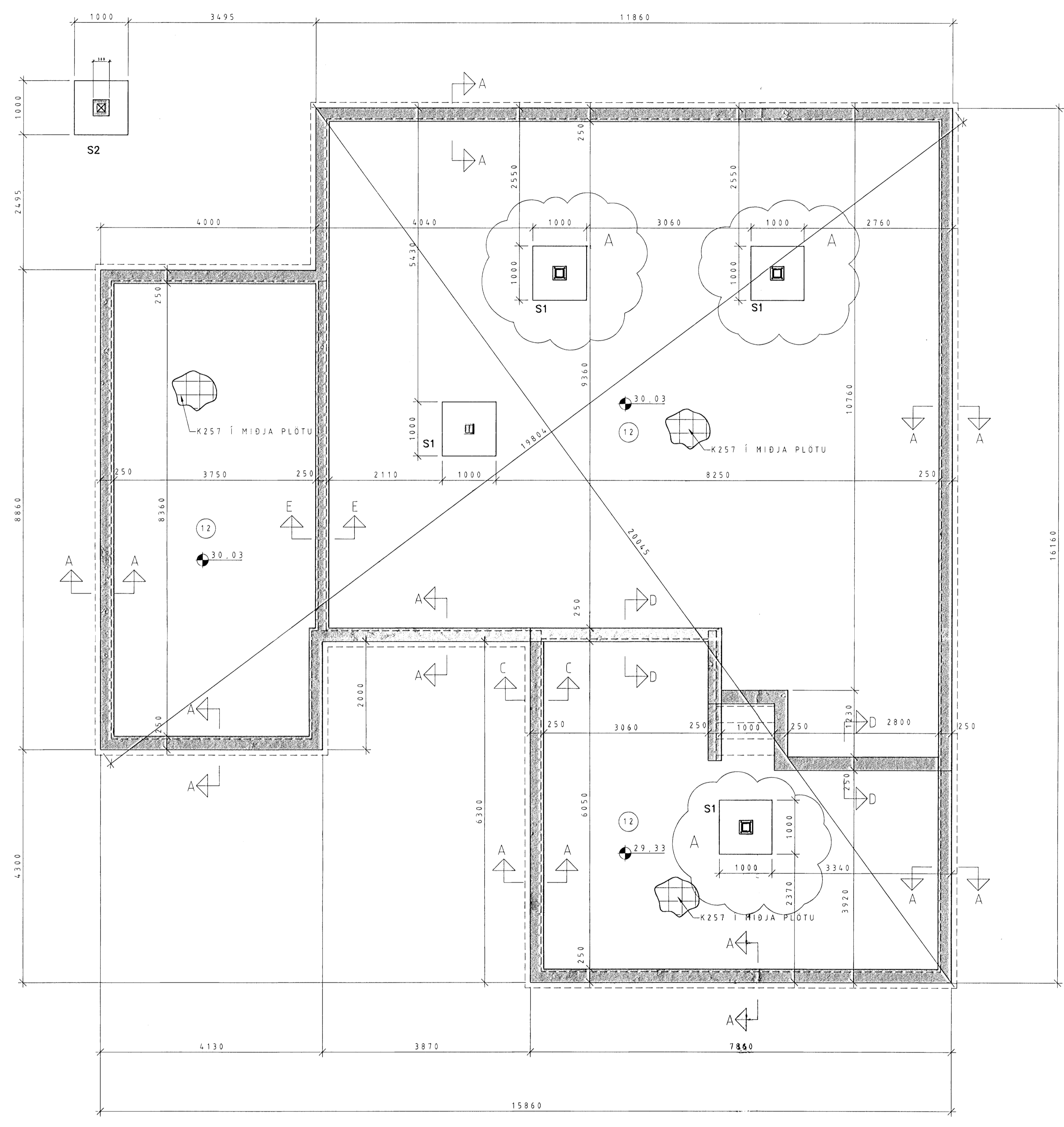
GRUNNMYND SÖKKLA 1 :50
