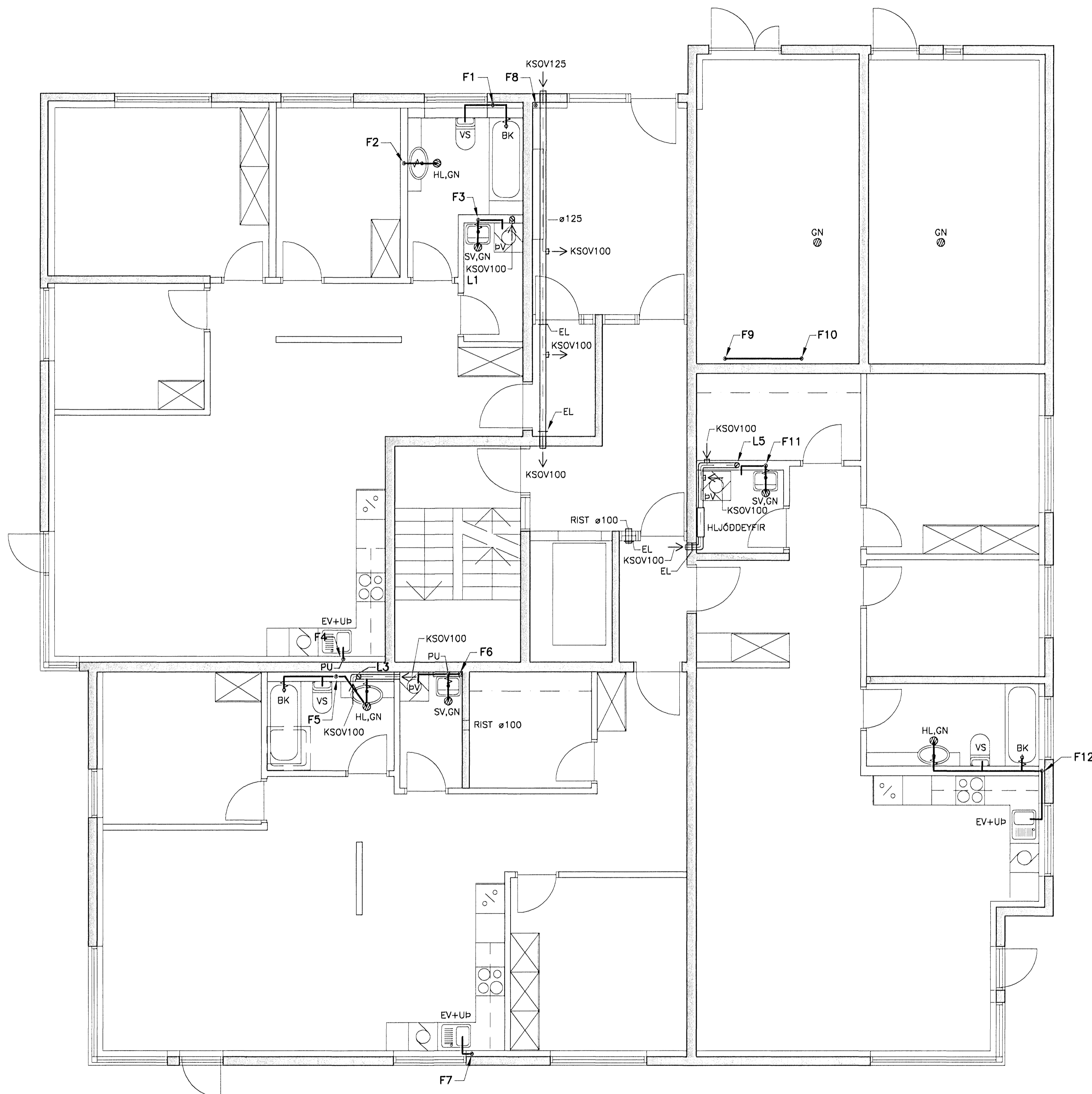
GRUNNMYND 1.HÆÐ, 1:50
