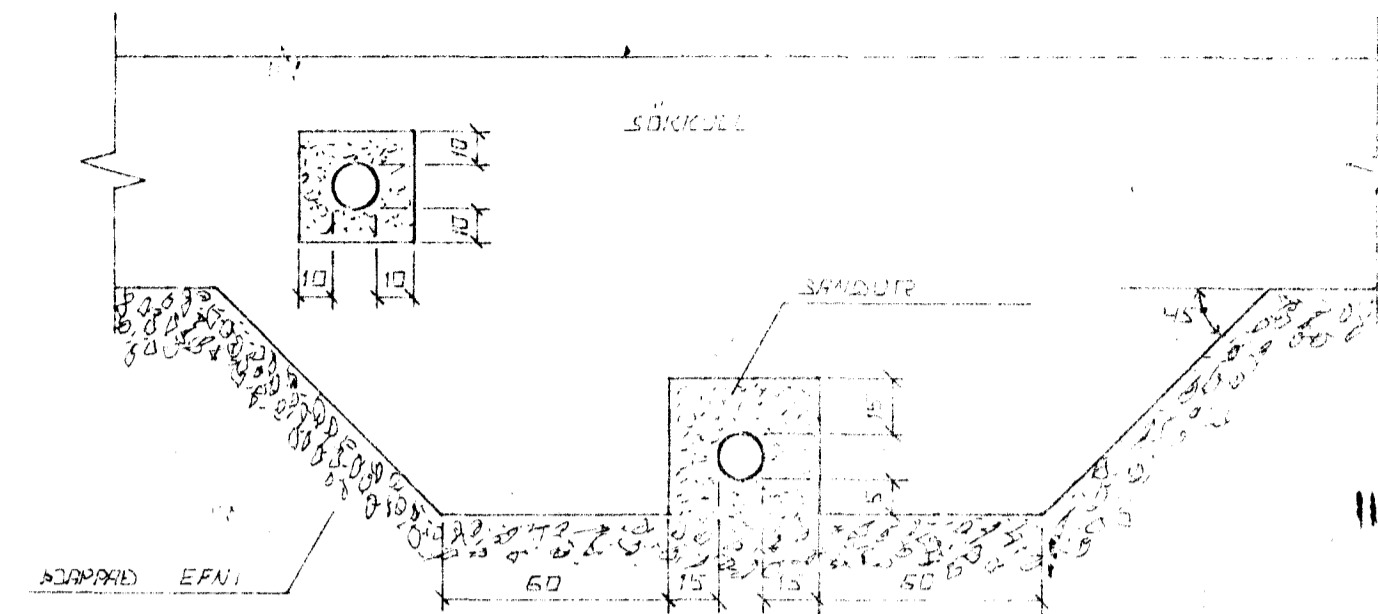
FRÁGANGUR LAGNA UNDIR DG Í SÖRKLÖÐ GRAFUR SKAL FÜRIR LÖGNUM UNDIR SÖRKLÖÐUM. AÐUR EN ÞEIR ERU STEIPTIR.
