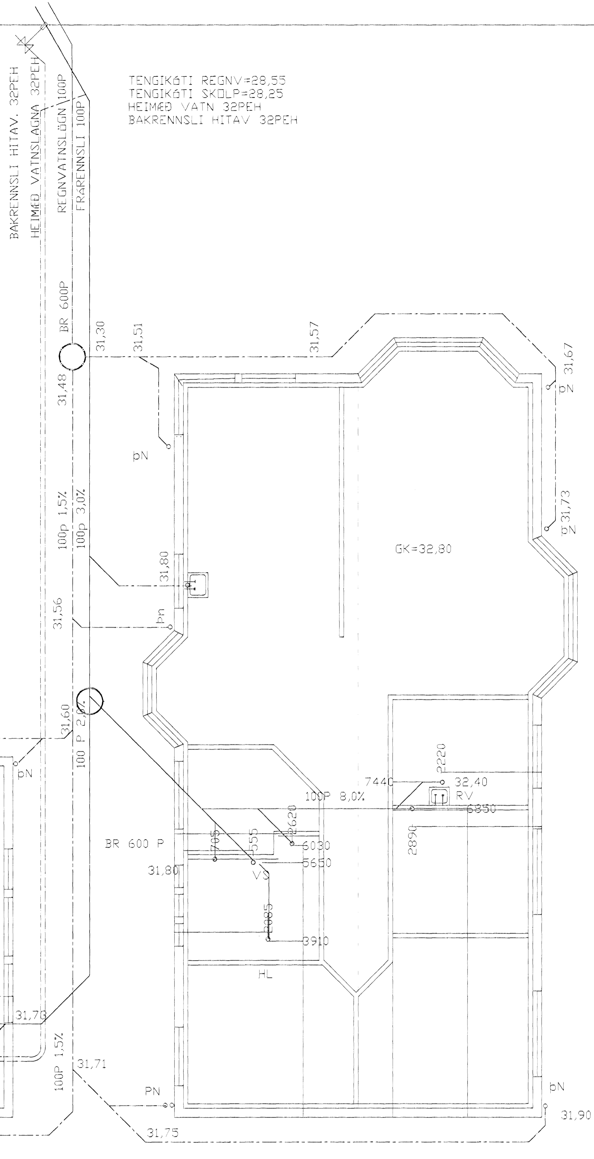
GRUNNMYND GRUNNLAGNIR 1/50
