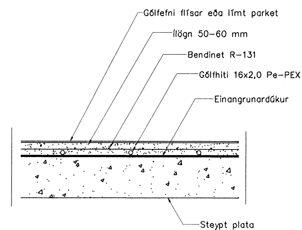
Gólfhiti snið, 1:10
