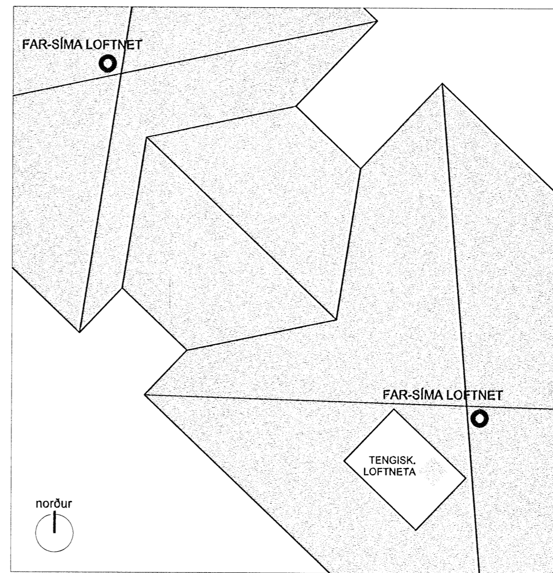
GRUNNMYND ÞAK mkv 1:100
