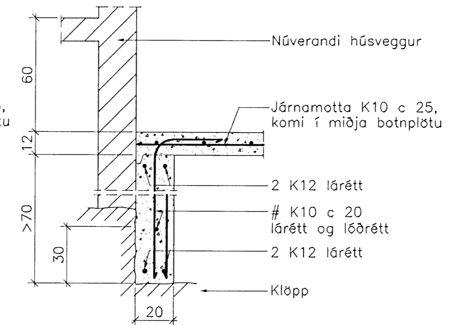
SNID D-D 1:20
