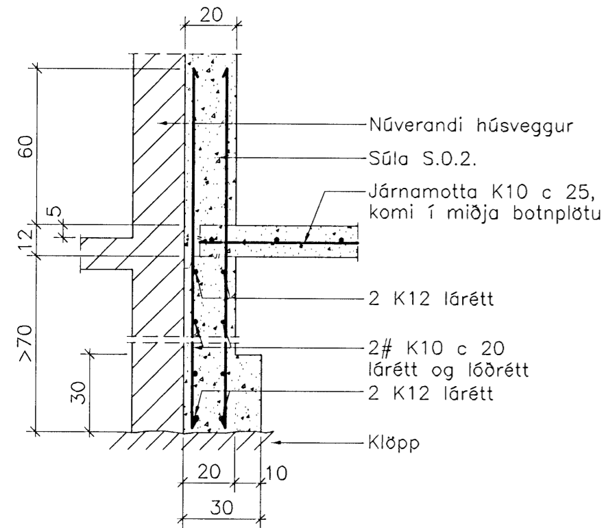
SNID A-A 1:20
