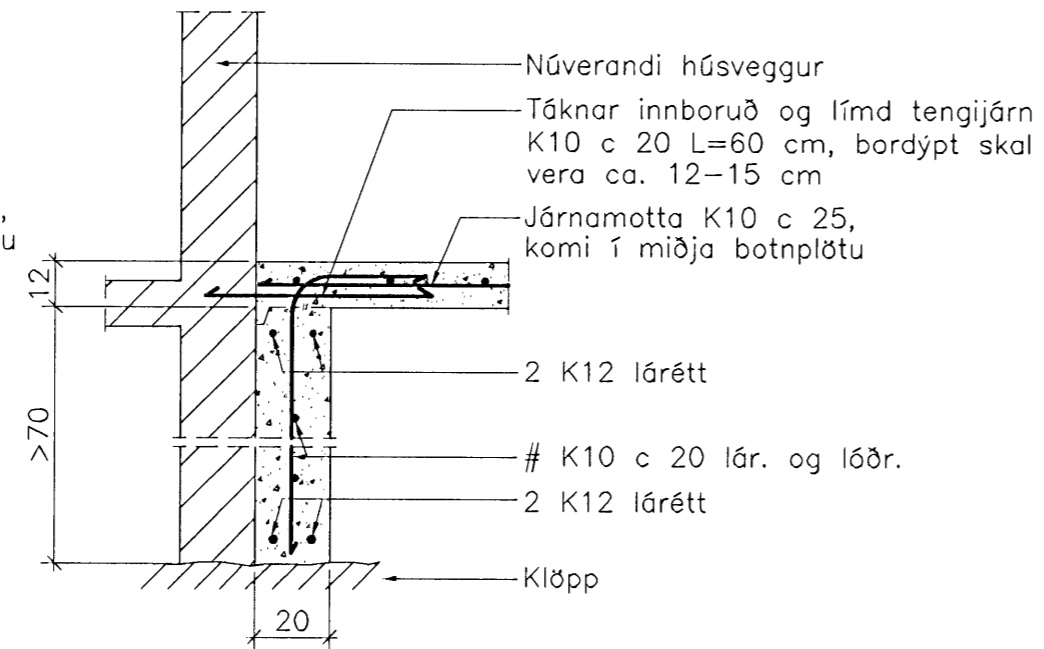
SNID B-B 1:20
