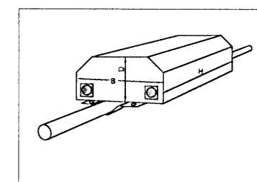
FAR-SÍMA LOFTNET STÆRÐ LOFTNETS: HxBxD=1309x167x89,5mm
