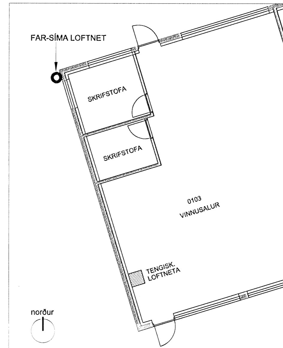
GRUNNMYND 1.HÆÐ mkv 1:100
