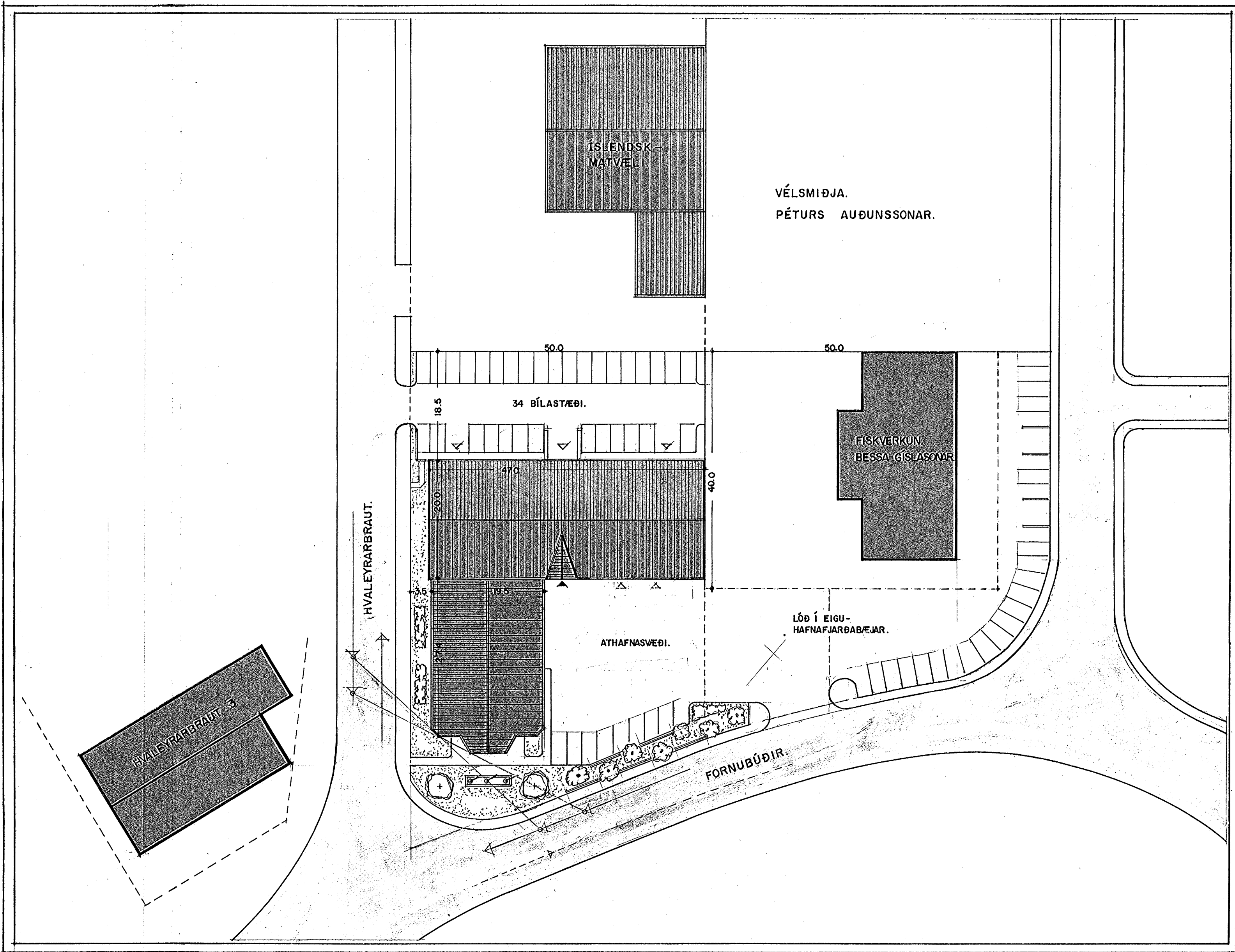
AFSTÓÐUMYND 1:500
