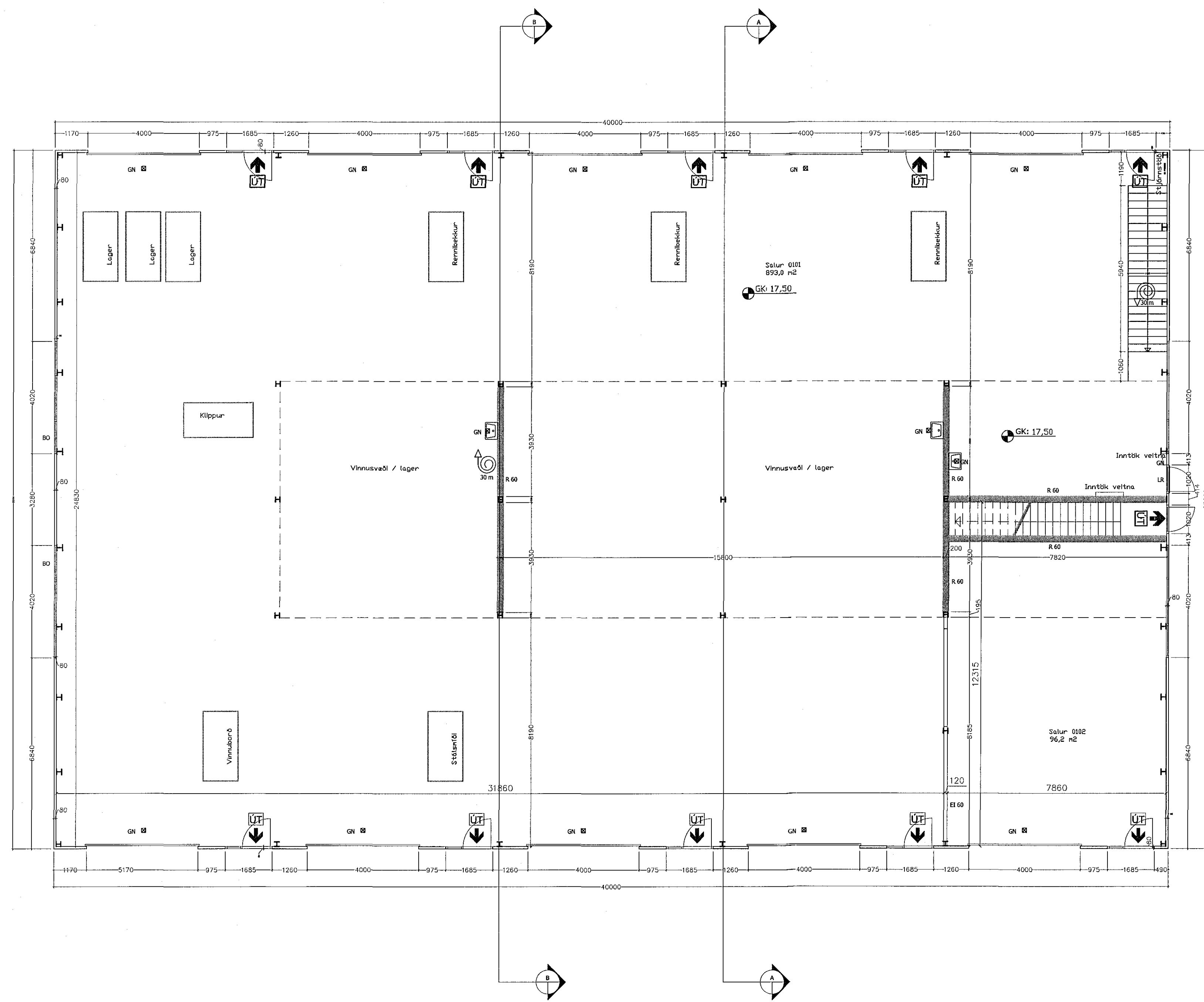
Grunnmynd 1. hæð
