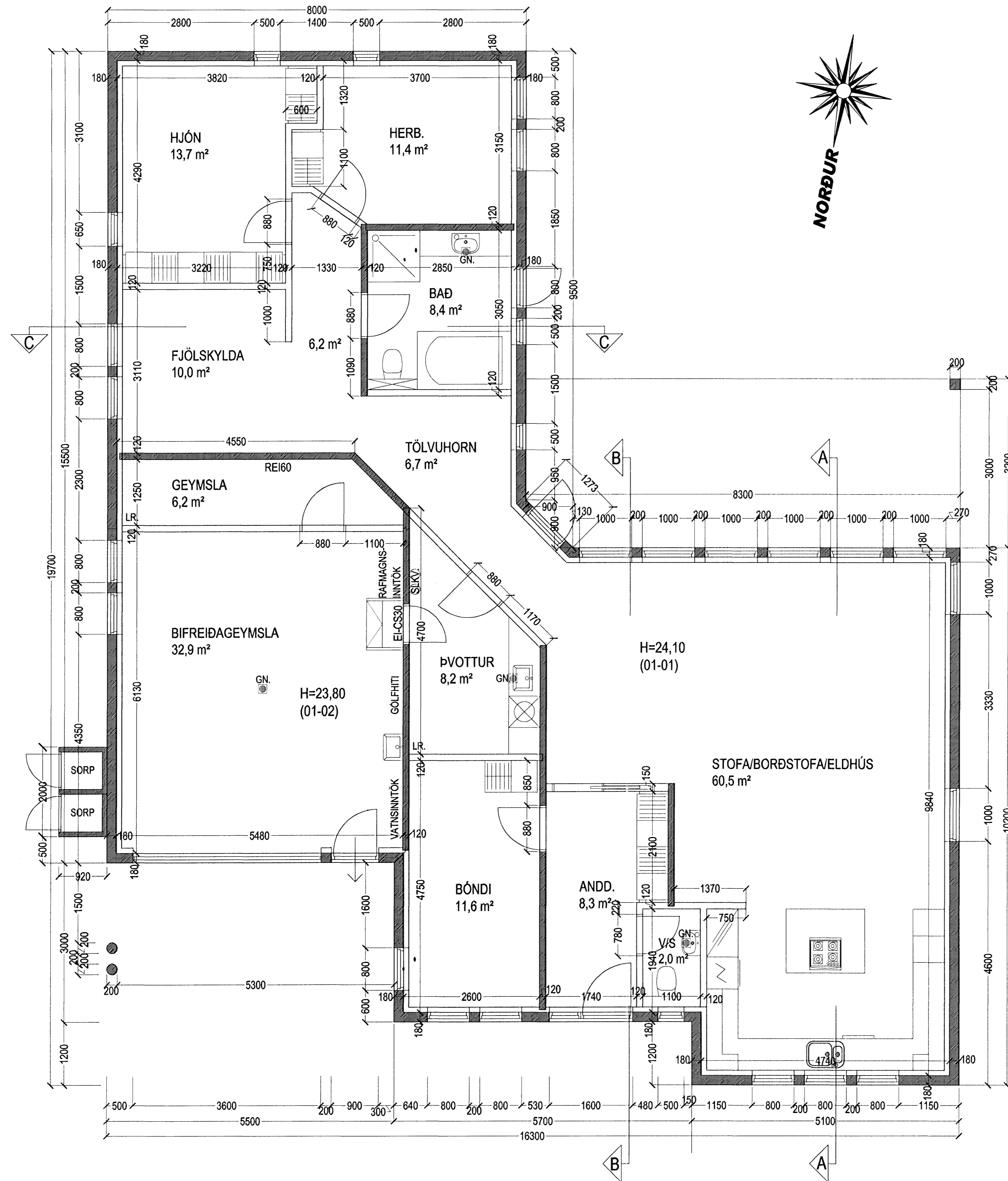
GRUNNMYND 1. HÆÐ MKV. 1:50.
