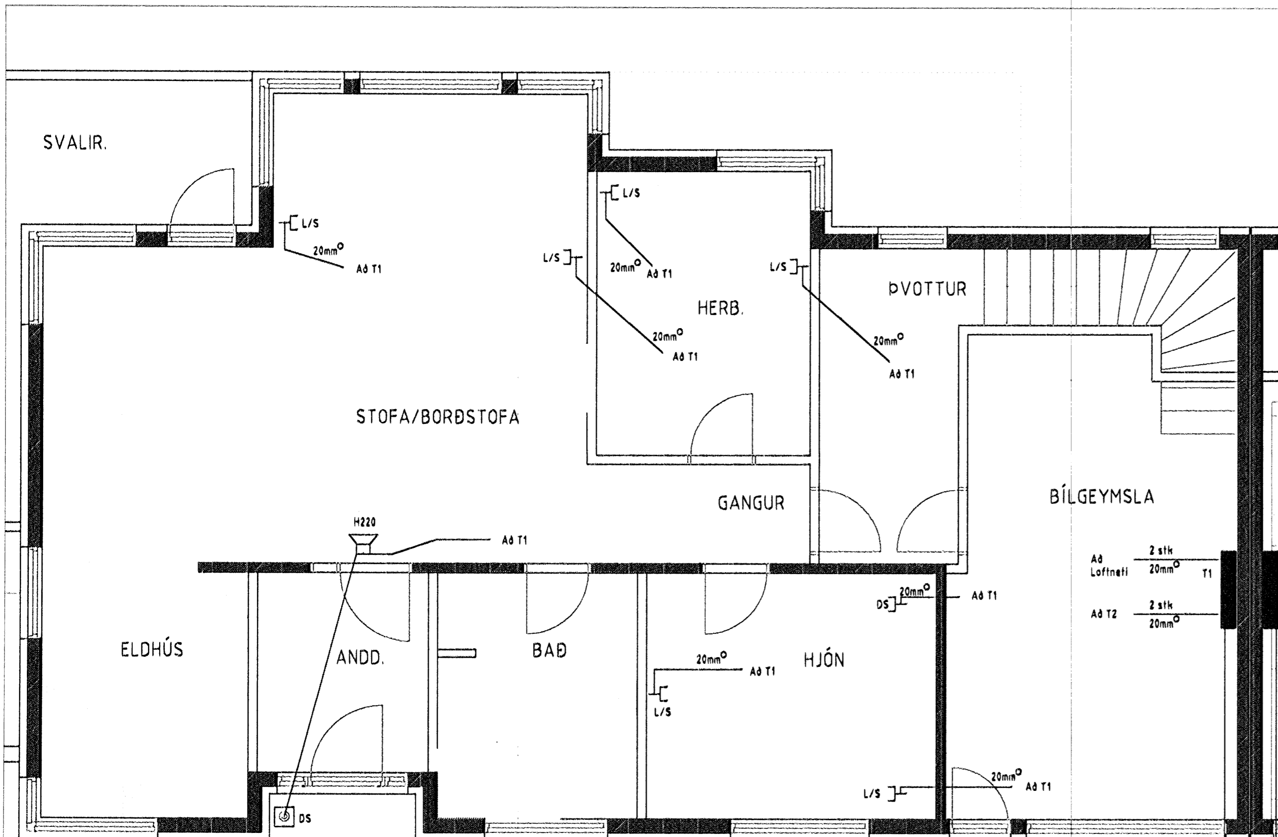
SMÁSPENNA HÆÐ MKV:1:50
