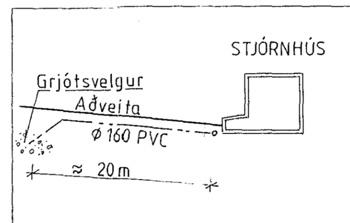
AFSTÖÐUMYND 1:500
