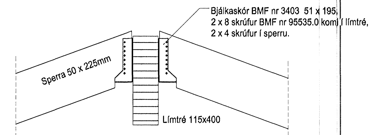
C Snið – Festing sperru á límtré Mkv. 1:10
