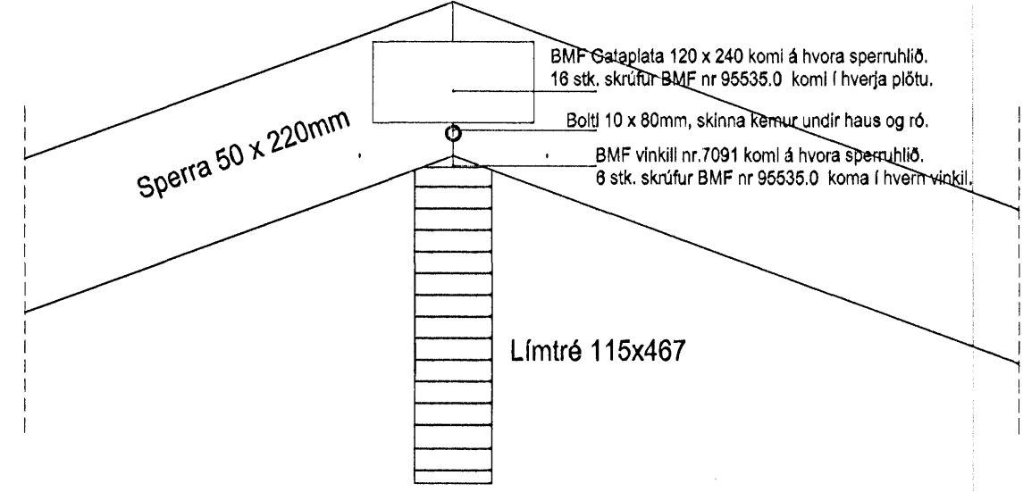
B Snið – Festing sperru á límtré Mkv. 1:10
