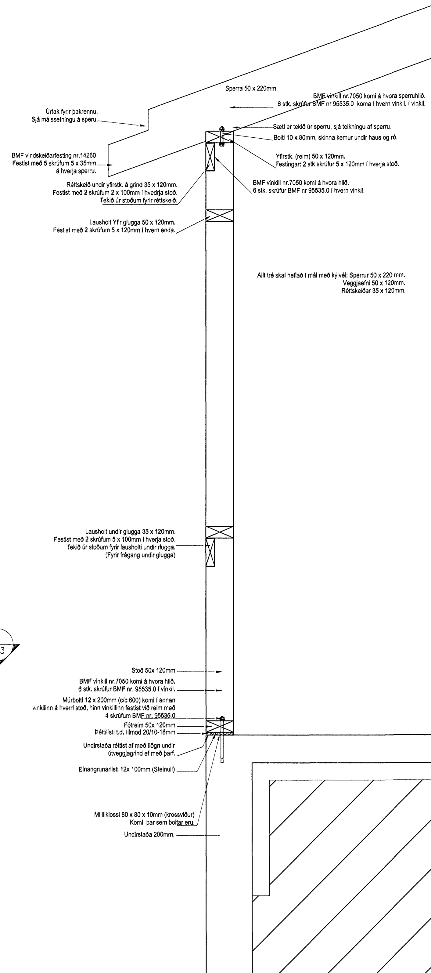
A Snið – Mkv. 1:10
