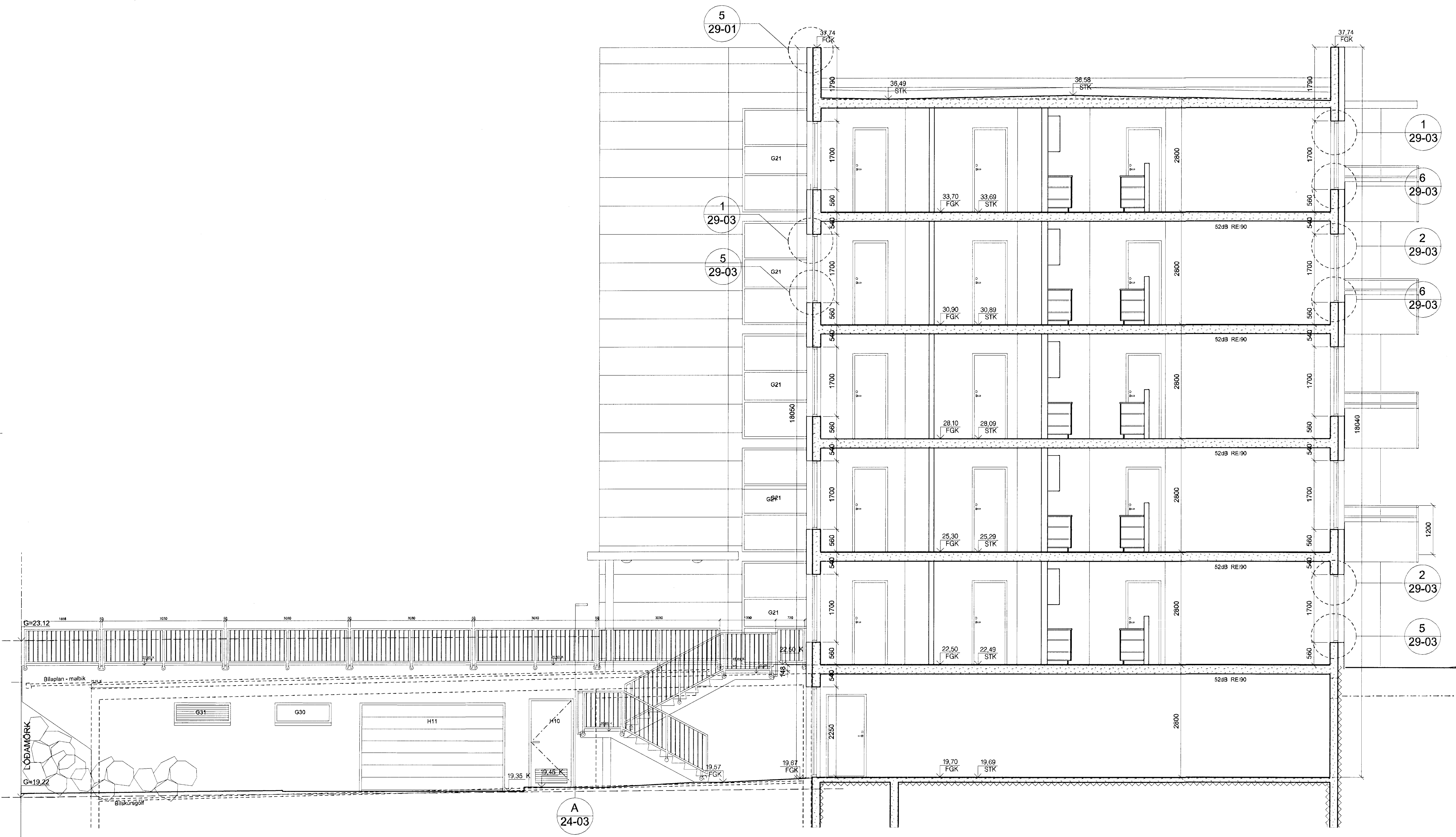
D-D 20-01 20-03 20-05 20-07 20-09 20-11 20-13 SNEIÐING 1:50
