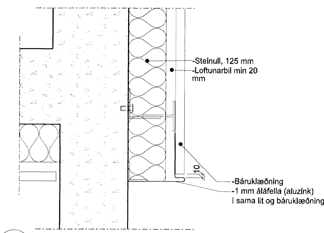
11 DEILI 1:5 BÁRA, LOKUN Á EINANGRUN
