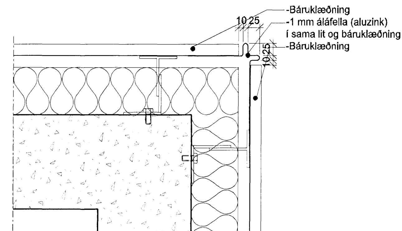
2 DEILI 1:5 ÚTHORN, BÁRA/BÁRA
