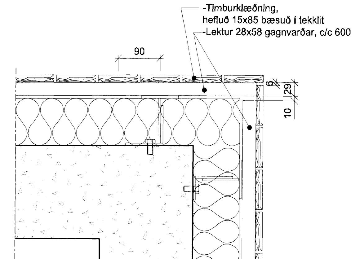
8 DEILI 1:5 ÚTHORN, VIÐUR/VIÐUR
