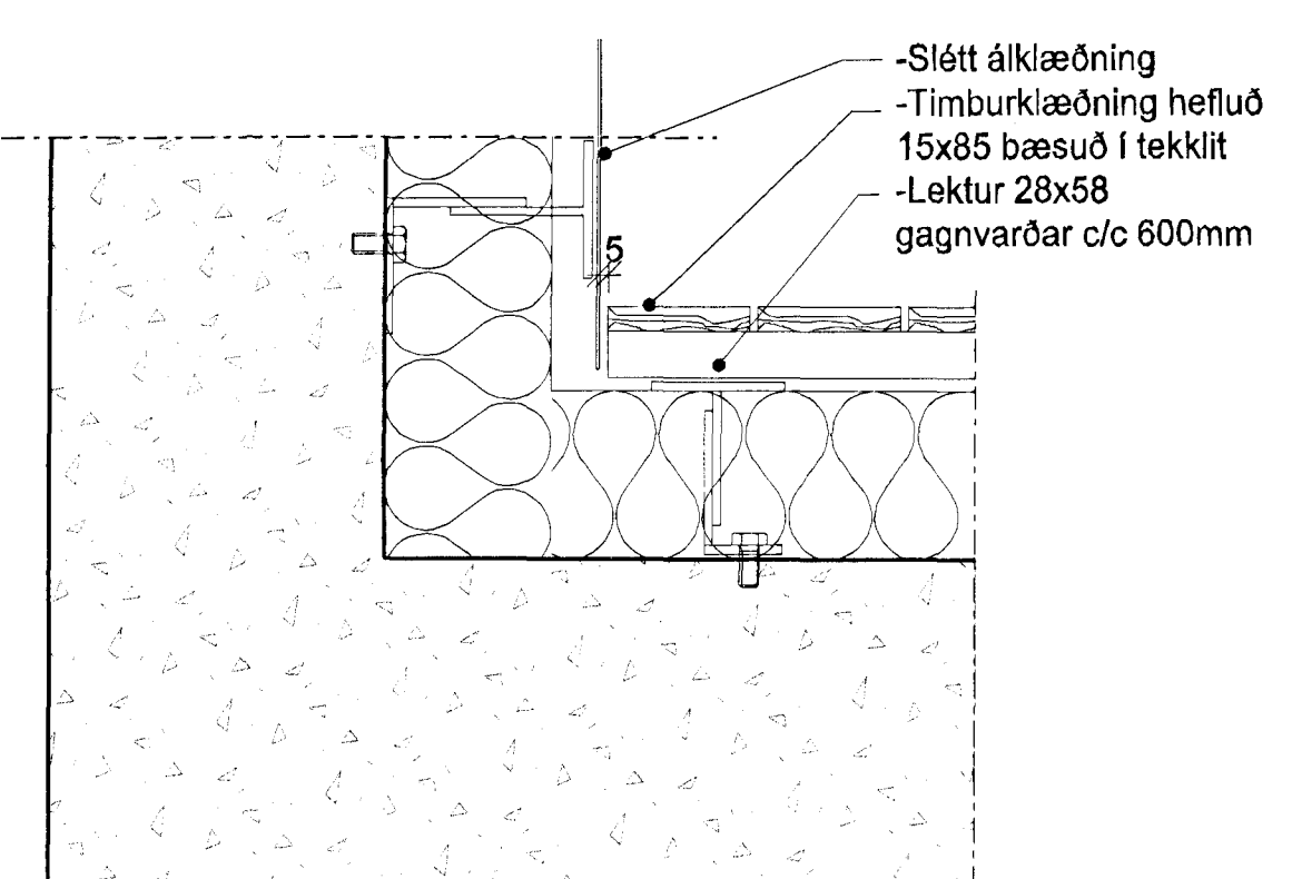
4 DEILI 1:5 INNHORN, SLÉTT/VIÐUR
